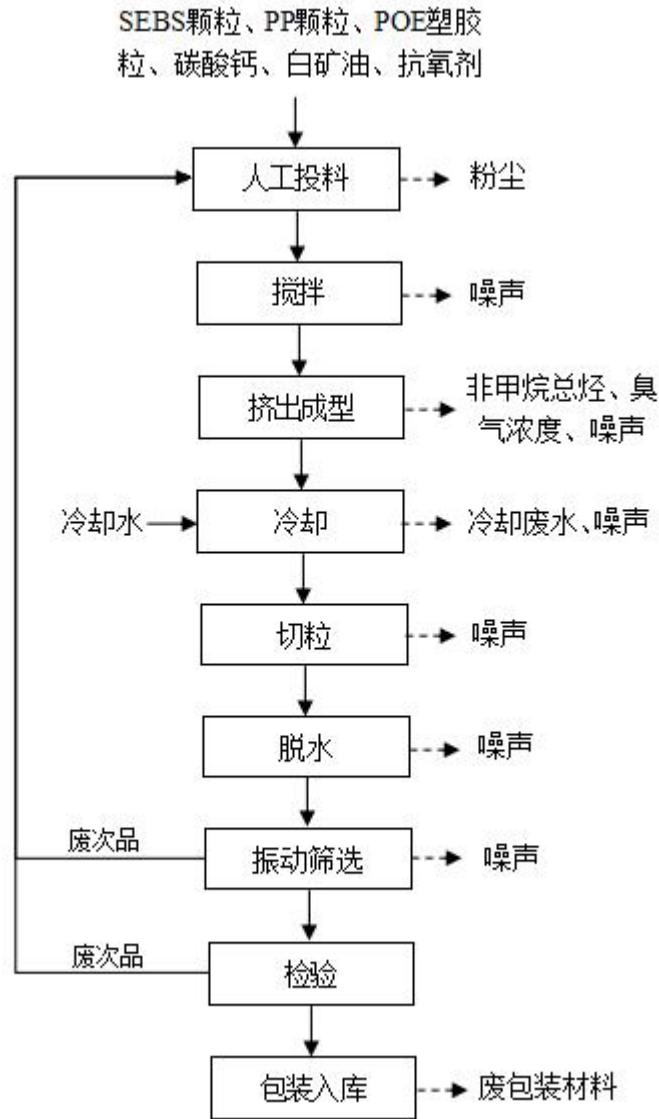
图 2-2 项目生产工艺流程图
