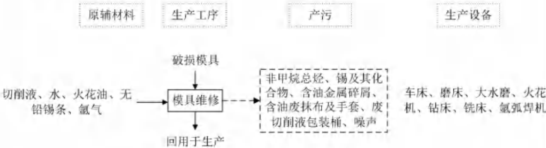
图 2-4 模具维修生产工艺流程图
