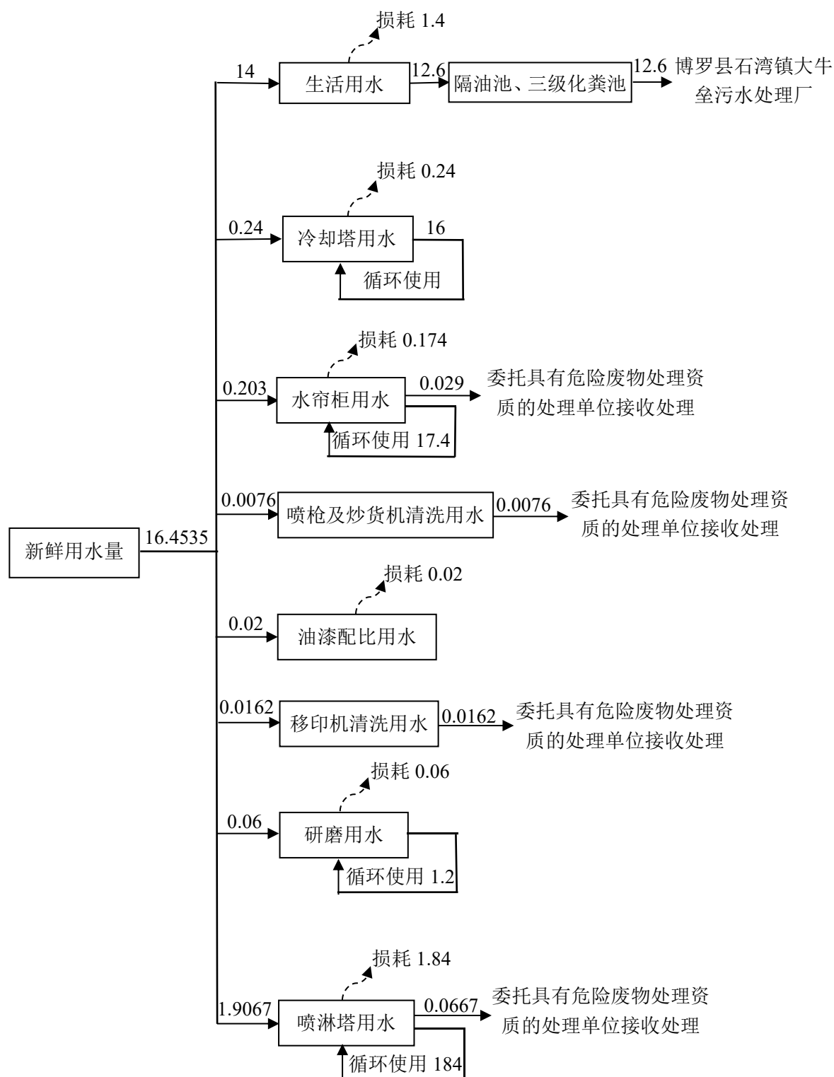
图 2-1 项目水平衡图 单位 t/d
