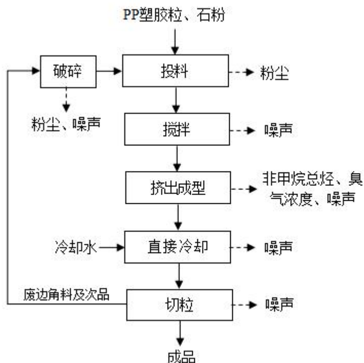
图 2-8 项目 PP 改性塑胶粒生产工艺流程及产污环节图
