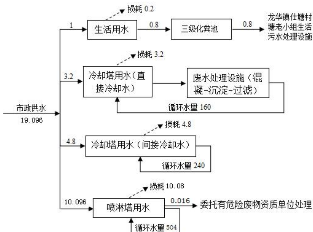
图 2-2 项目水平衡图 (t/d)
