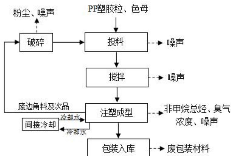
图 2-7 项目植草格生产工艺流程及产污环节图
