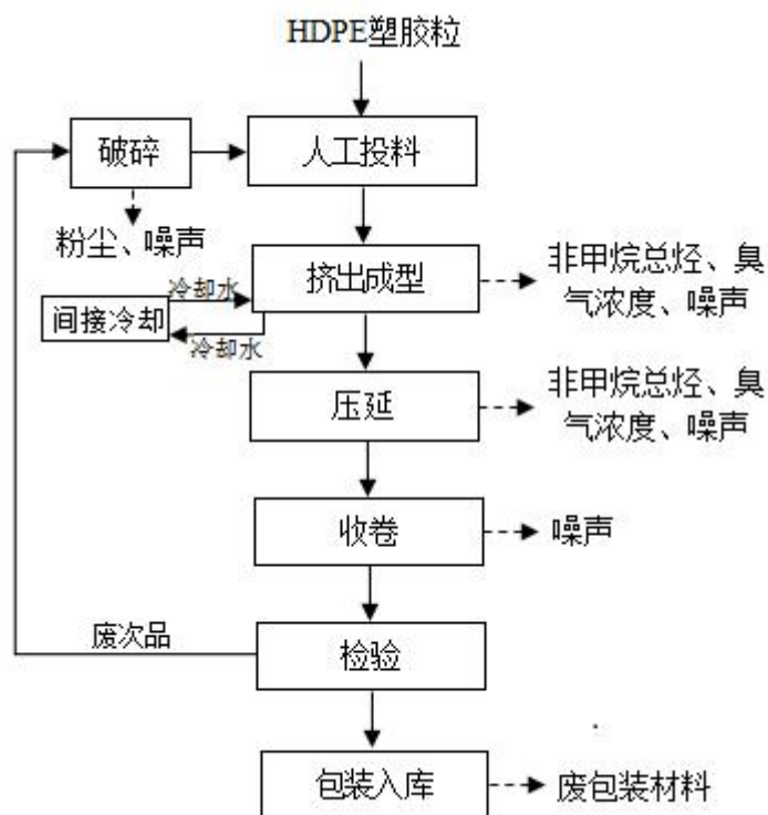
图 2-9 项目土工膜生产工艺流程及产污环节图
