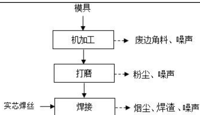
图 2-10 项目模具修理工艺流程及产污环节图
