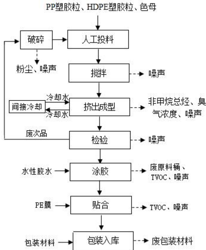
图 2-5 项目排水板生产工艺流程及产污环节图
