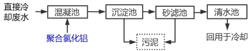
图 4-1 废水处理设施工艺流程图
