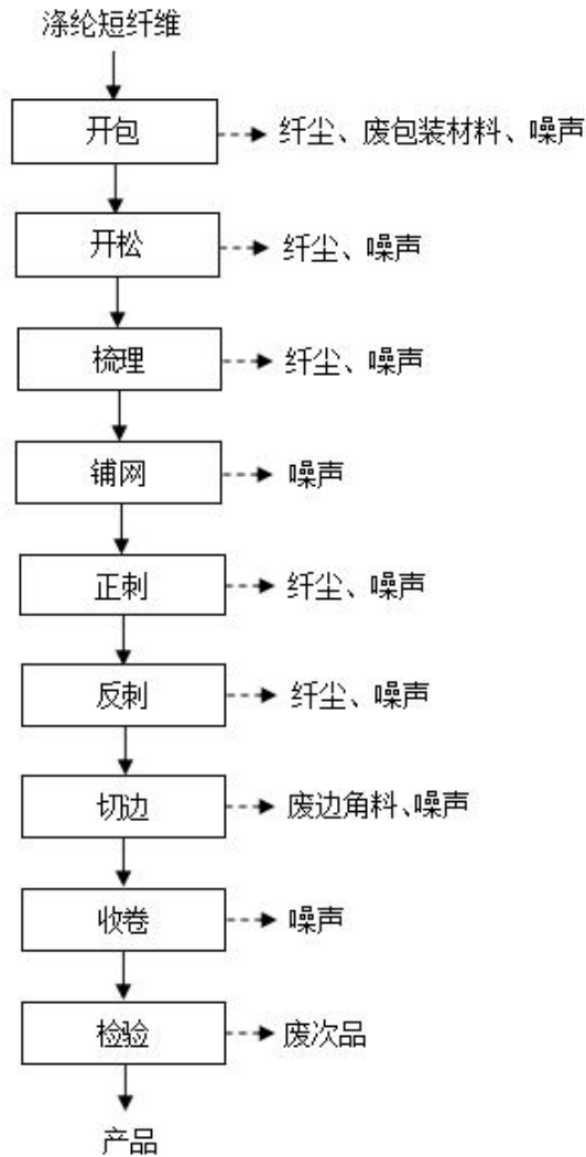
图 2-3 项目土工布生产工艺流程及产污环节图
