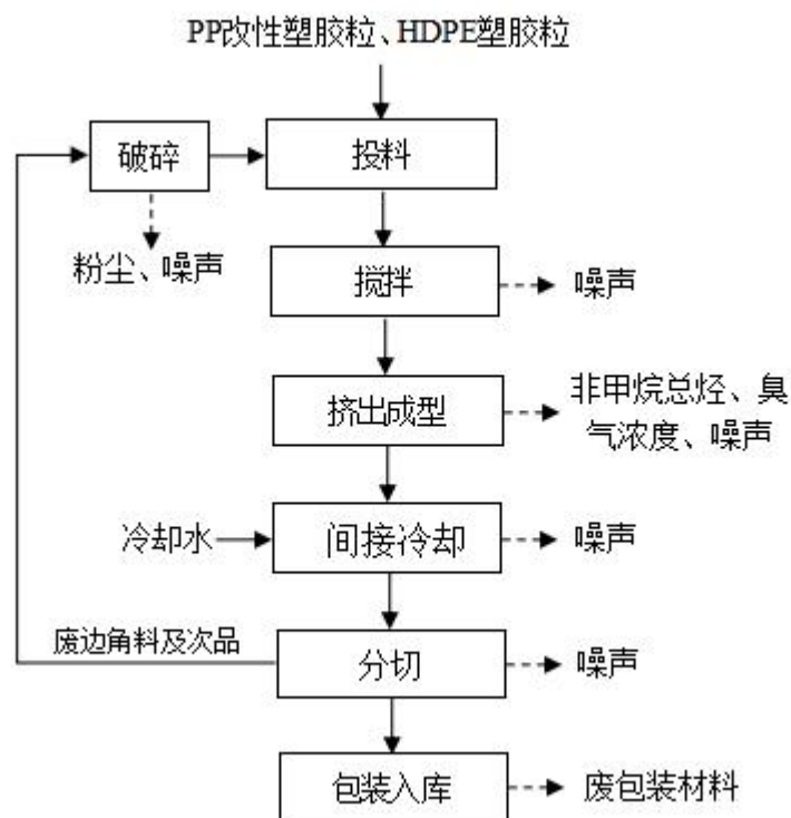
图 2-4 项目塑胶盲沟管、硬式透水管生产工艺流程及产污环节图
