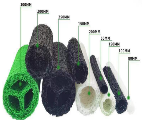
塑料盲沟管
