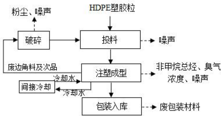
图 2-6 项目蓄排水板生产工艺流程及产污环节图
