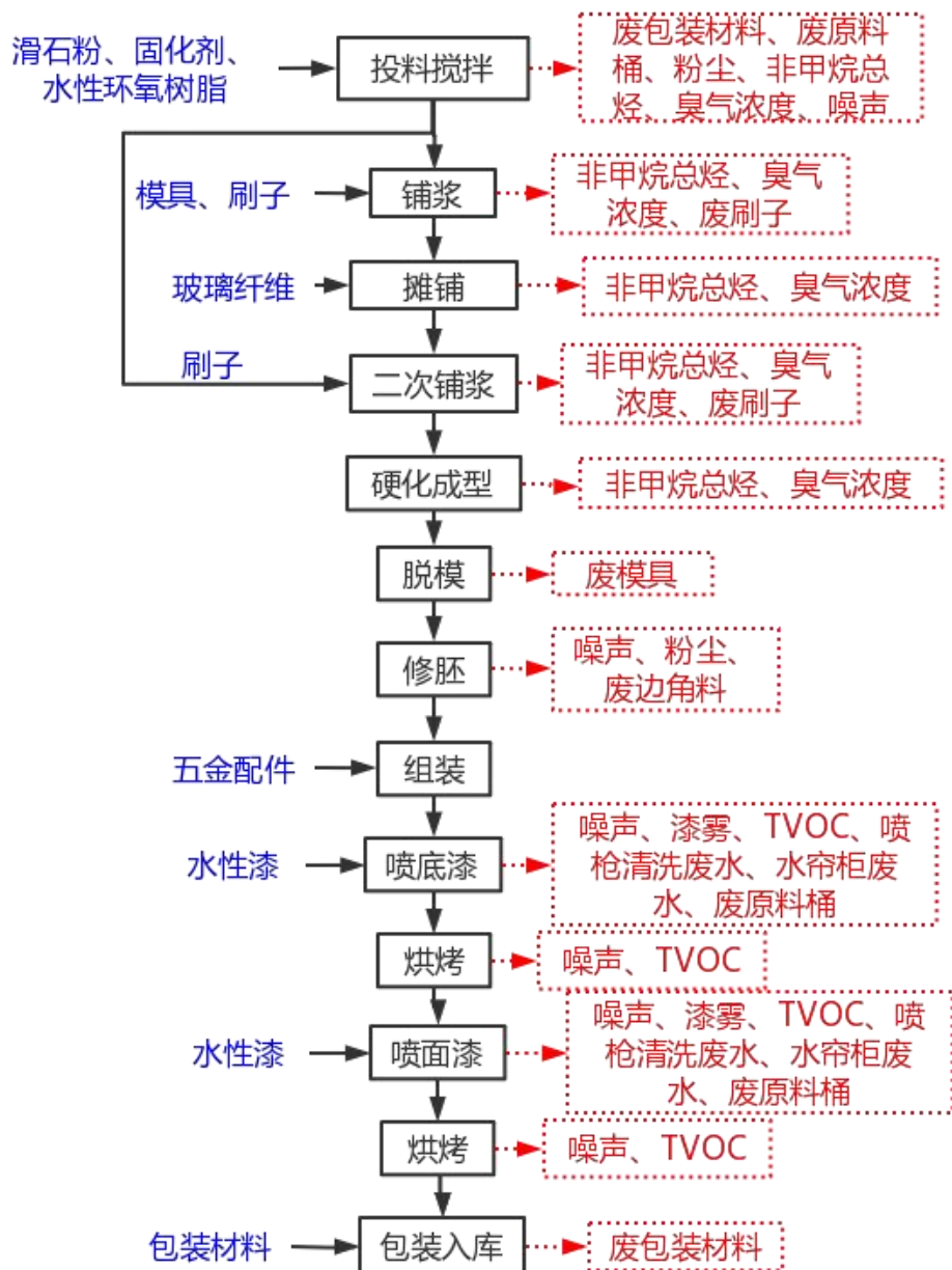
图 2-2 项目工艺流程及产污环节图
