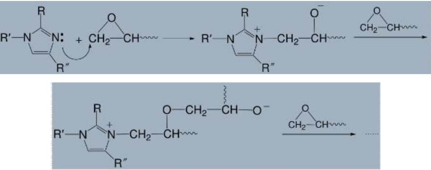
图 2-3 咪唑类固化剂与环氧树脂固化原理
