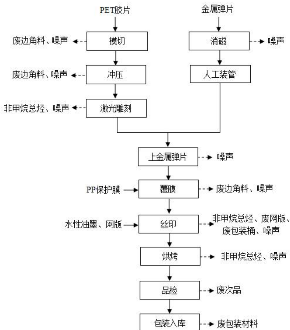
图2-1 项目工艺流程及产污环节图
