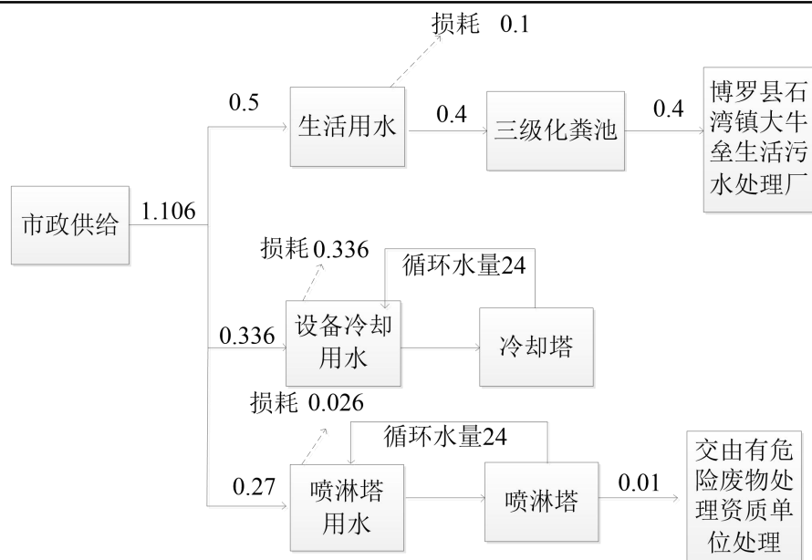
图1 项目水平衡图
