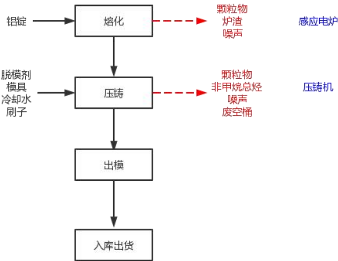
图 2-4 自行车车架生产工艺流程图
