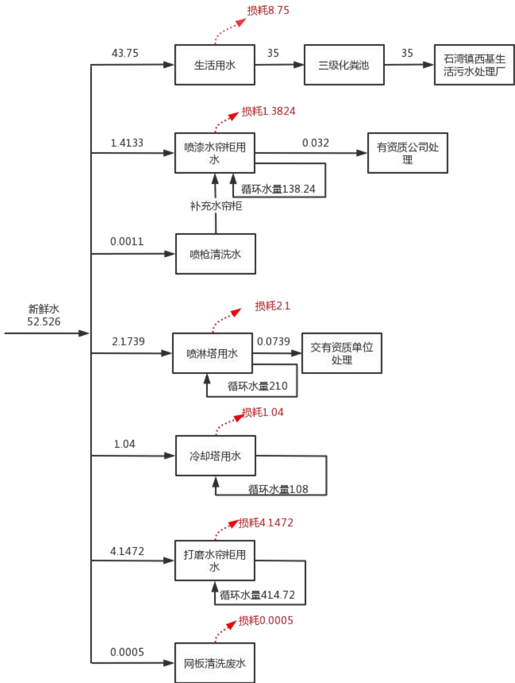
图 2-3 项目水平衡图 单位 t/d
