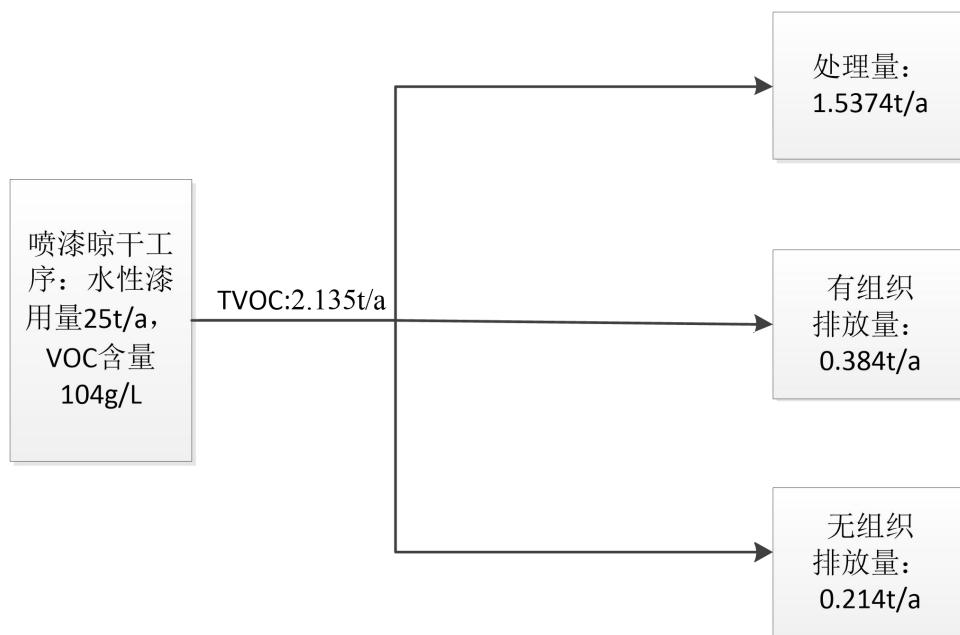
图 2-1 生产项目 VOCs 平衡图
