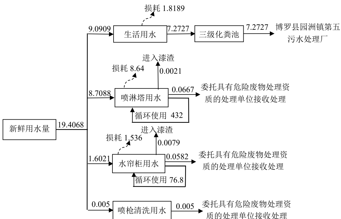
图 2-2 项目水平衡图 单位 t/d
