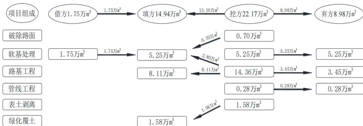
图 2-3 土石方平衡图
