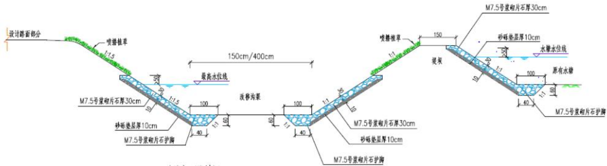
图 2-4 K1+100~K1+356、K2+020~K2+440 路段改沟断面设计图
