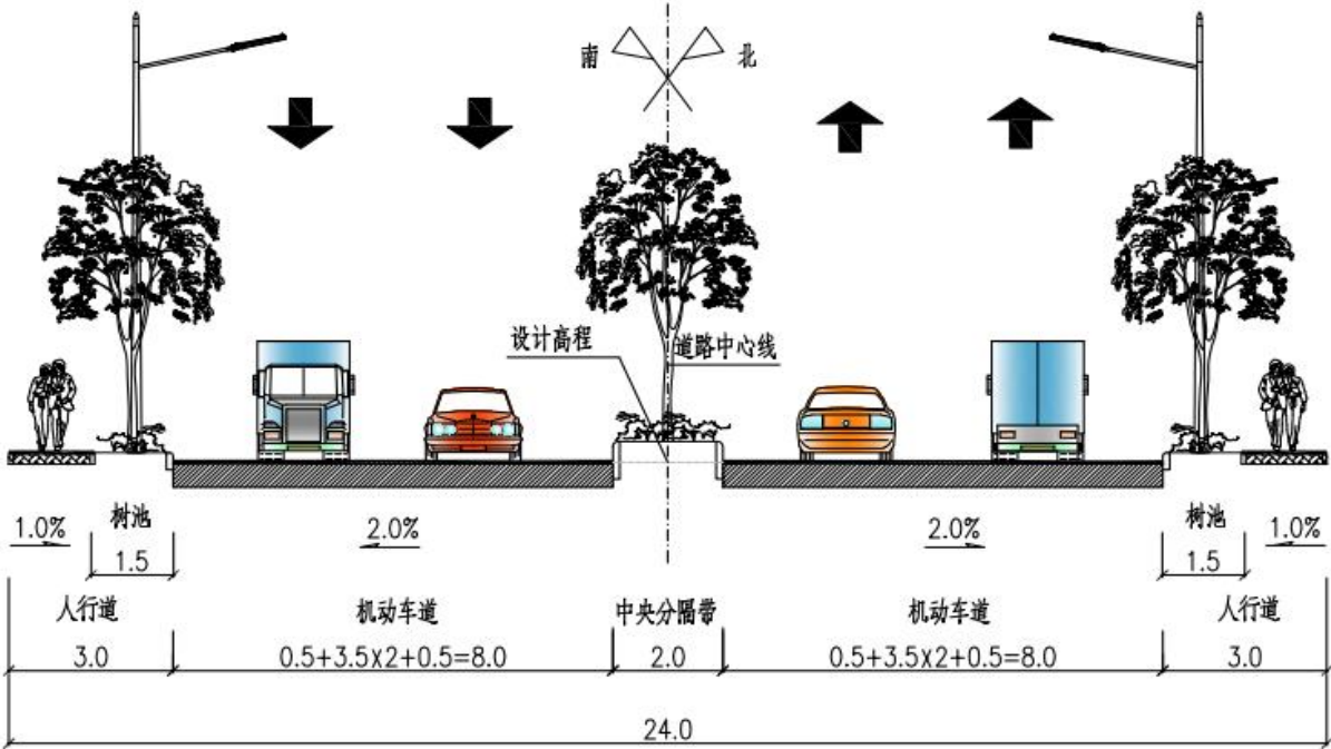
图 2-1 道路横断面布置图
