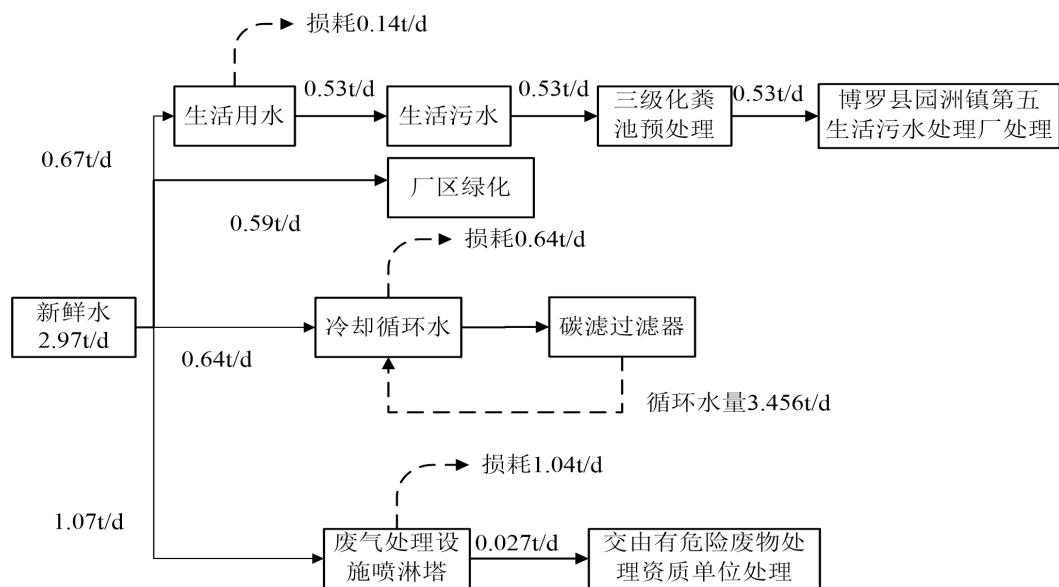
图2-1a 远期项目水平衡图 (t/d)
