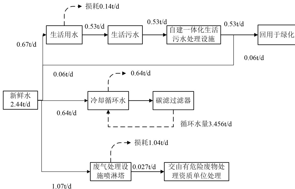
图2-1b 近期项目水平衡图 (t/d)
