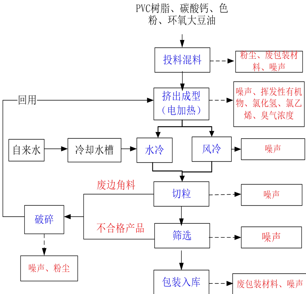
图2-2 工艺流程图
