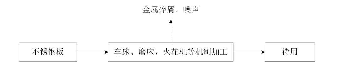
图 2-6 现有项目模具生产工艺流程及产污节点示意图
