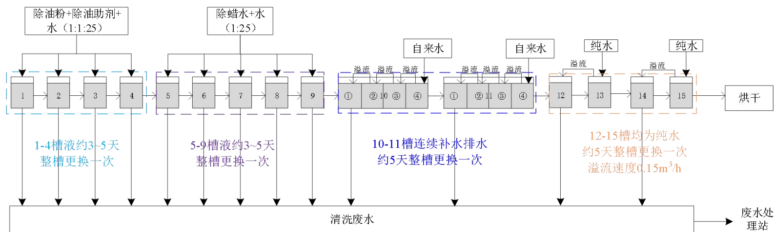
图2-3 超声波清洗流程示意图
