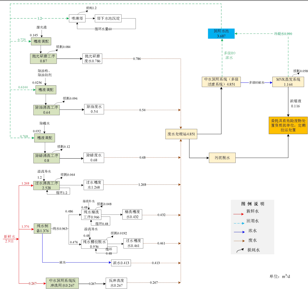
图 2-1 改扩建项目水平衡图
