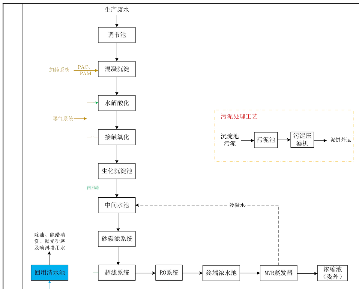
图 4-1 项目废水处理工艺
