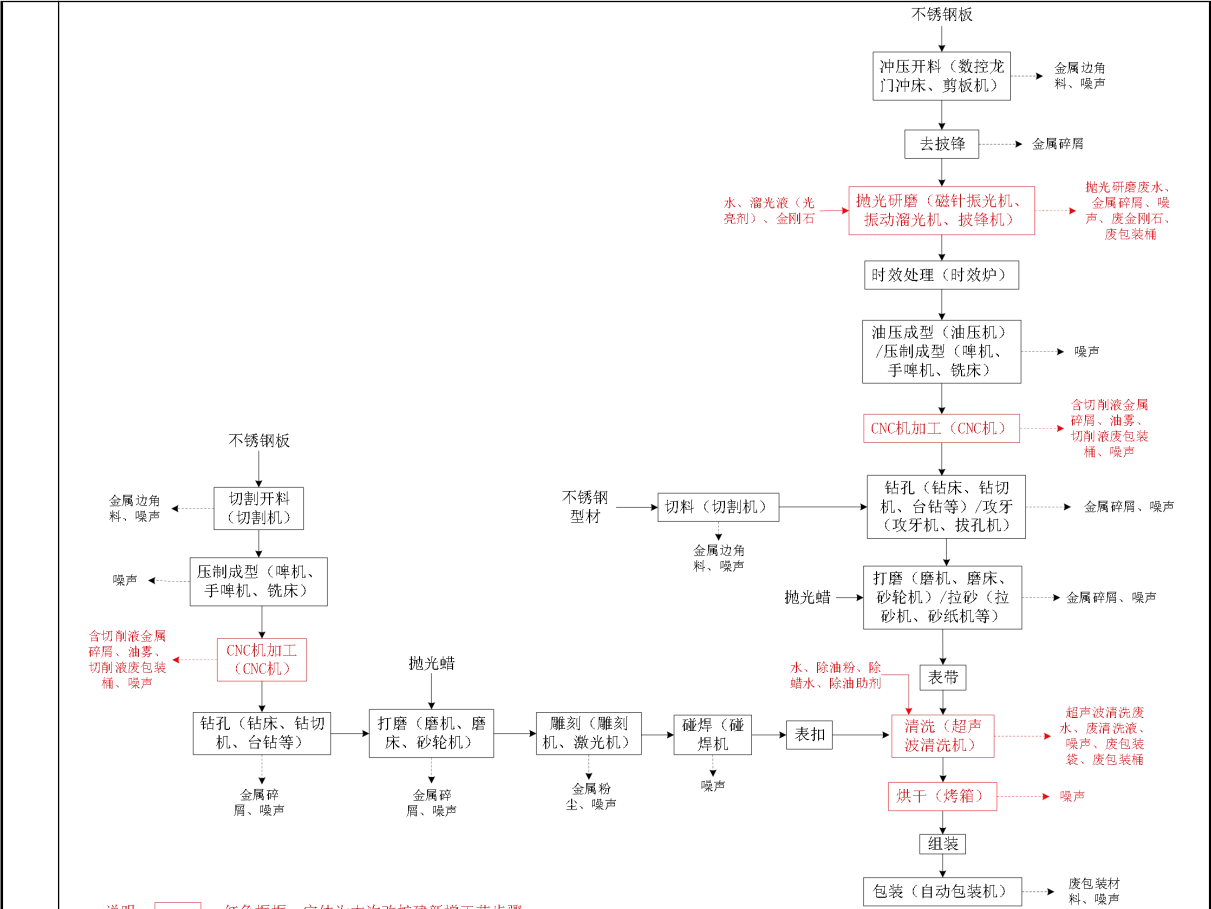
图 2-4 改扩建项目表带生产工艺流程及产污节点示意图
