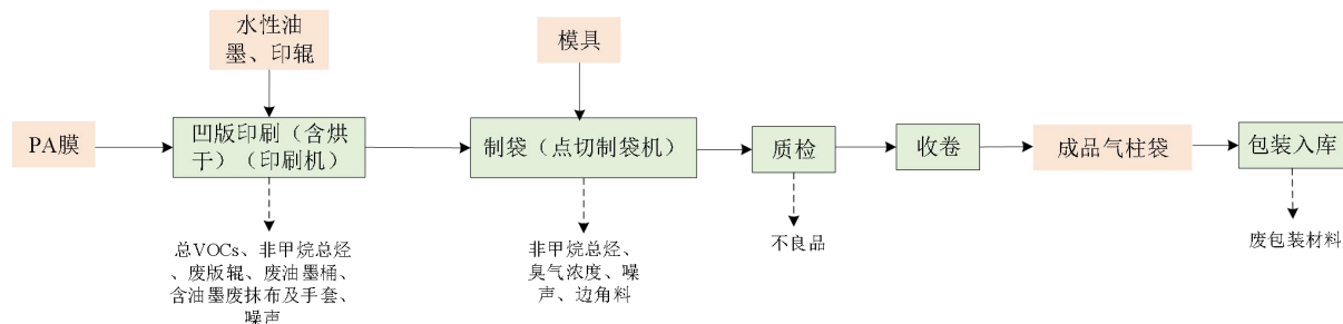
图3 气柱袋生产工艺流程及产污节点示意图
