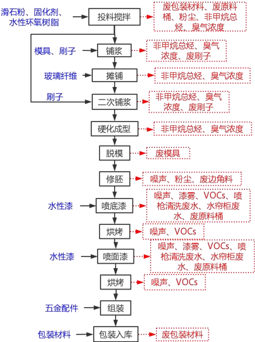
图 2-2 项目工艺流程及产污环节图
