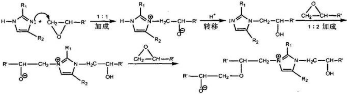
图2-3 咪唑类固化剂与环氧树脂固化原理
