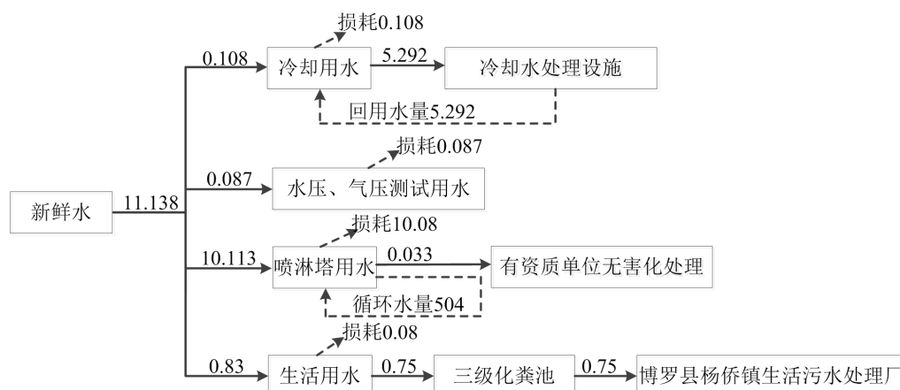
图 2-1 项目营运期间水平衡图 (m³/d)
