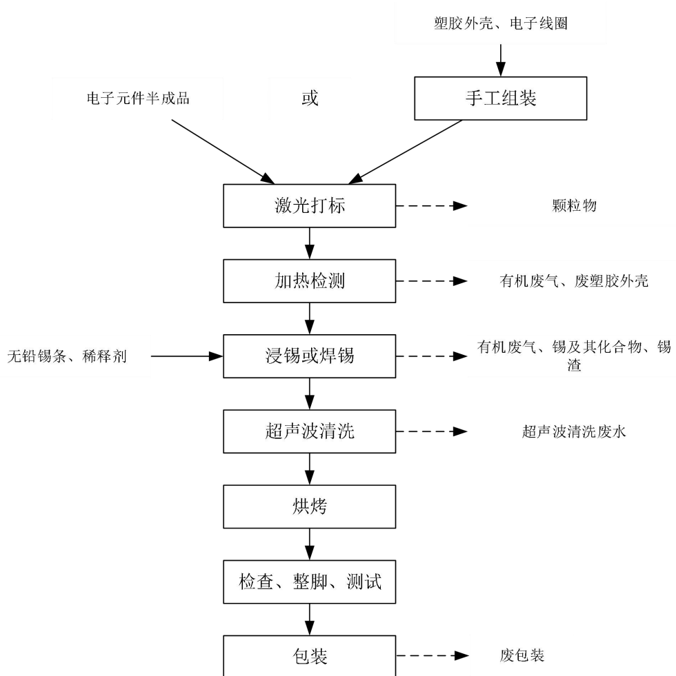
图 2-3 项目网络变压器生产工艺流程图
