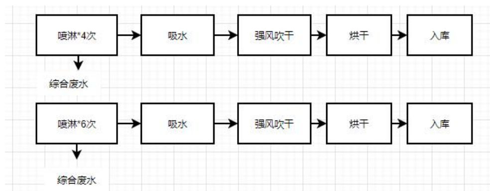
图 2-9 改扩建后新增清洗线工艺流程
