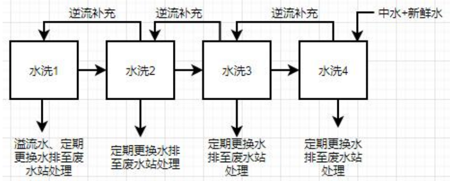
图 2-10 清洗线 1 的水洗流程图
