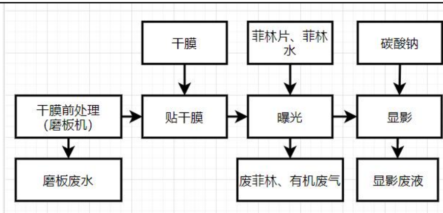
图 2-8 改扩建后图形转移工艺流程图
