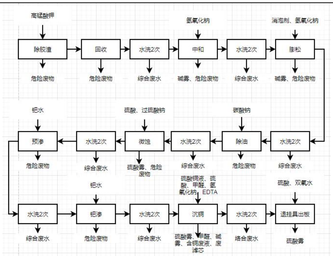
图 2-3 改扩建后项目沉铜线主要生产工艺流程图
