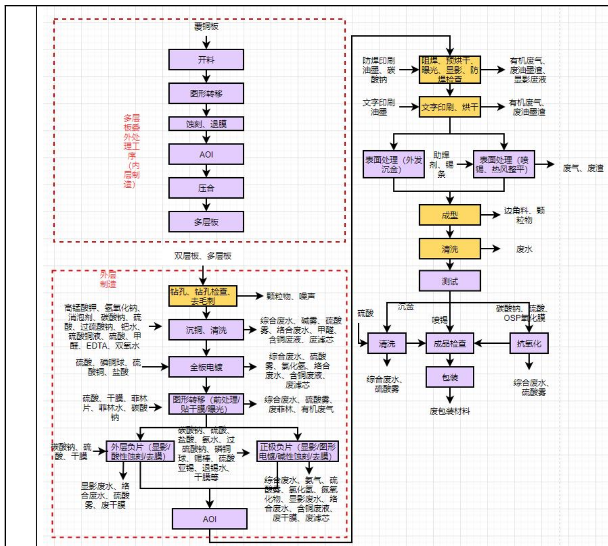
图 2-2 改扩建项目双面板、多层板生产工艺流程及产污节点图
