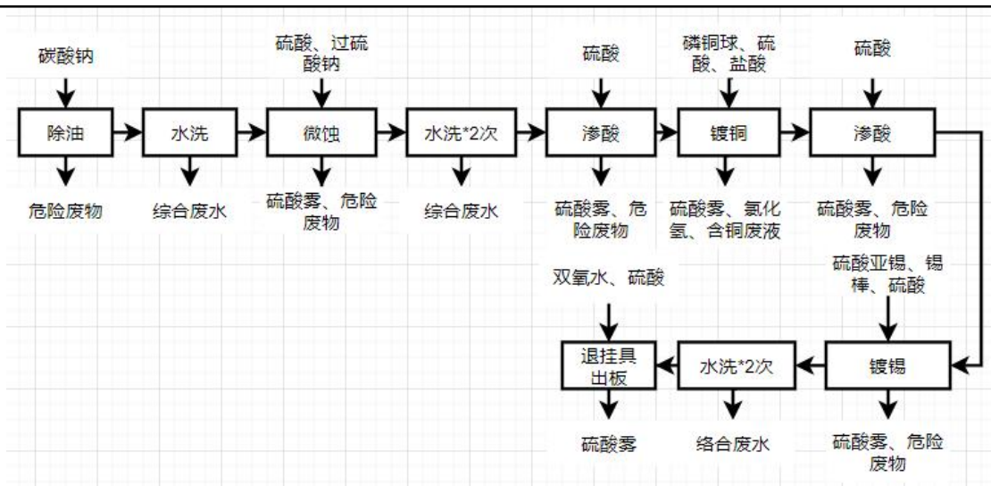
图 2-4 改扩建后项目图形电镀线工艺流程图
