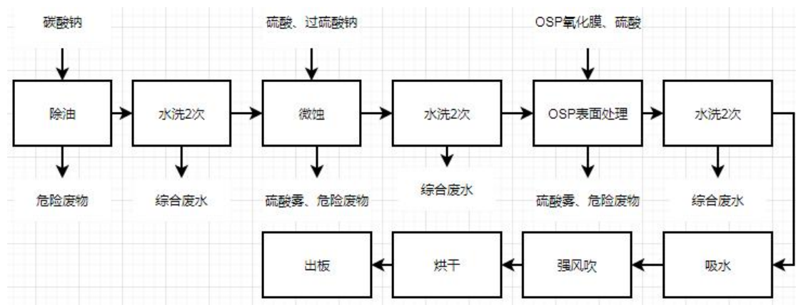
图 2-7 改扩建后 OSP 表面处理线工艺流程图
