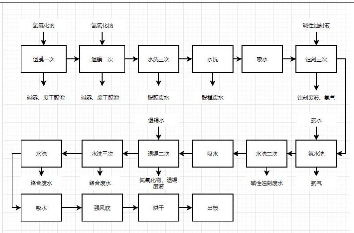
图 2-6 改扩建后项目蚀刻线工艺流程
