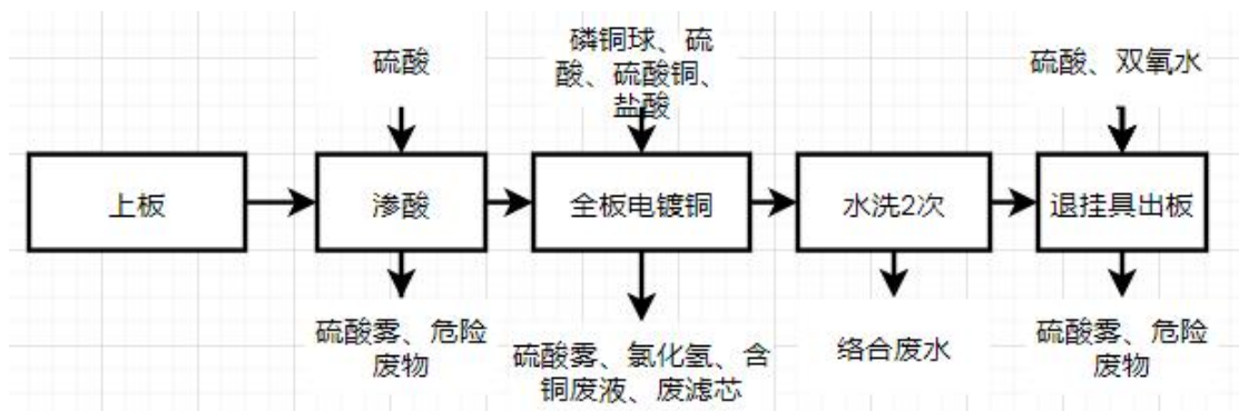
图 2-5 改扩建后项目全板电镀线工艺流程
