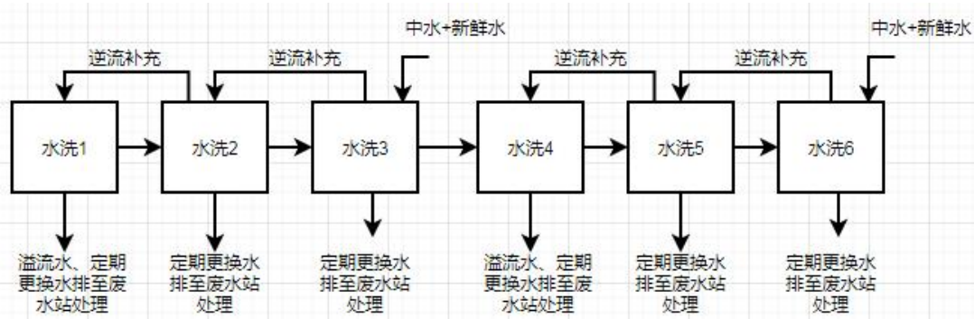
图 2-11 清洗线 2 的水洗流程图
