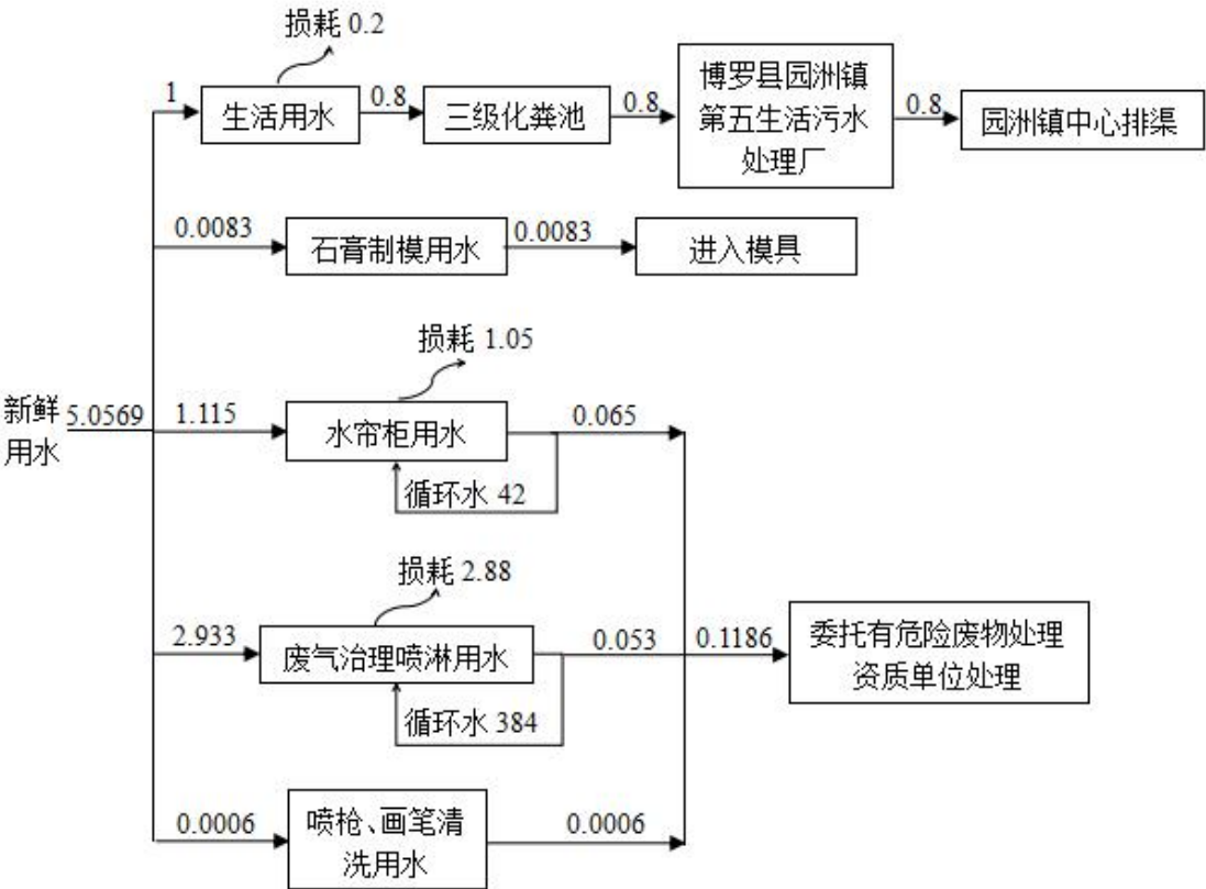
图 2-1 项目用水平衡图（单位 t/d）
