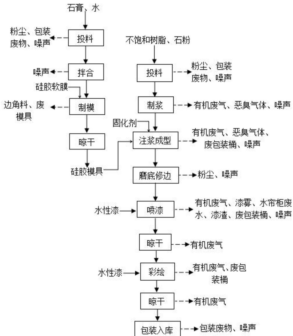
图 2-1 项目生产工艺流程
