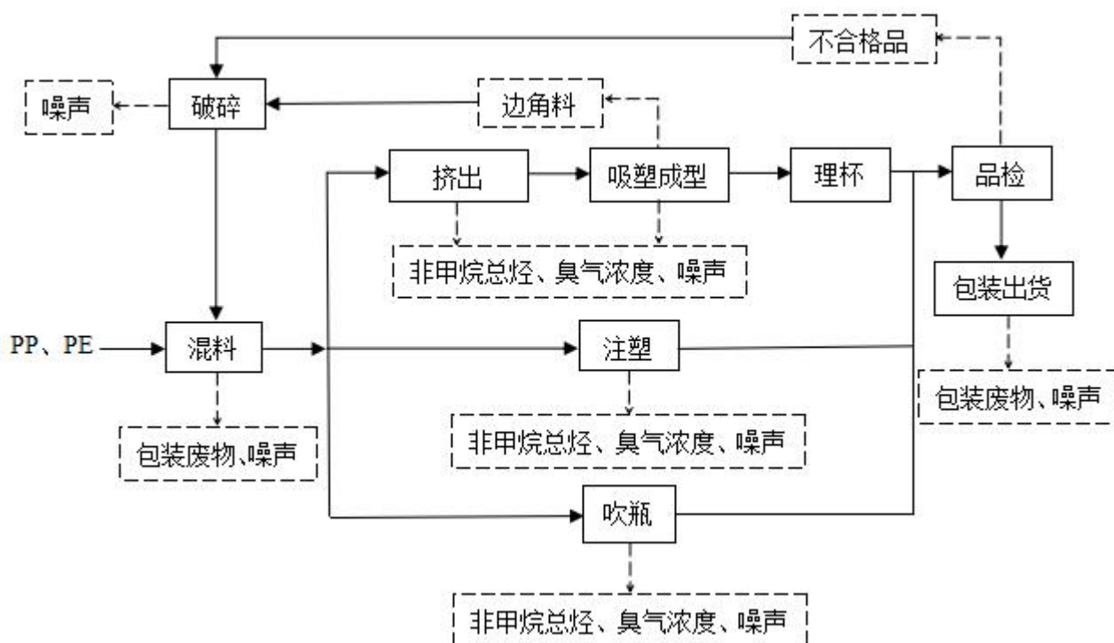
图 2-1 项目生产工艺流程
