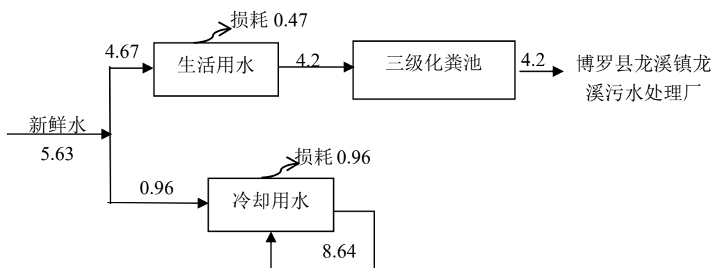
图 2-1 现有项目水平衡图 (t/d)
