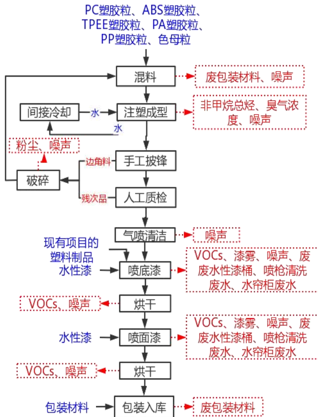
图 2-4 项目生产工艺流程图
