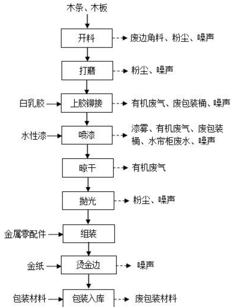
图 2-2 项目生产工艺流程及产污环节图
