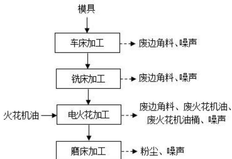
图 2-5 项目模具修理工艺流程及产污环节图
