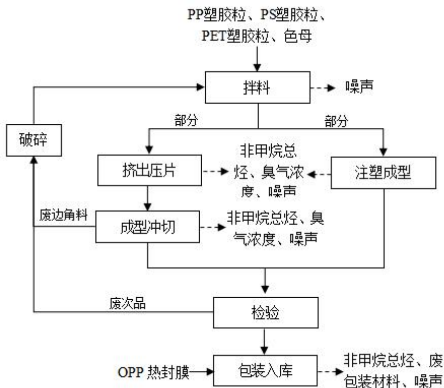
图 2-3 项目盖子生产工艺流程图
