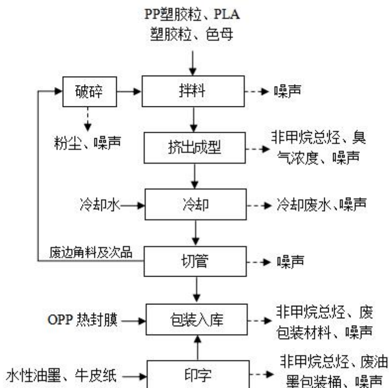
图 2-4 项目杯子生产工艺流程图
