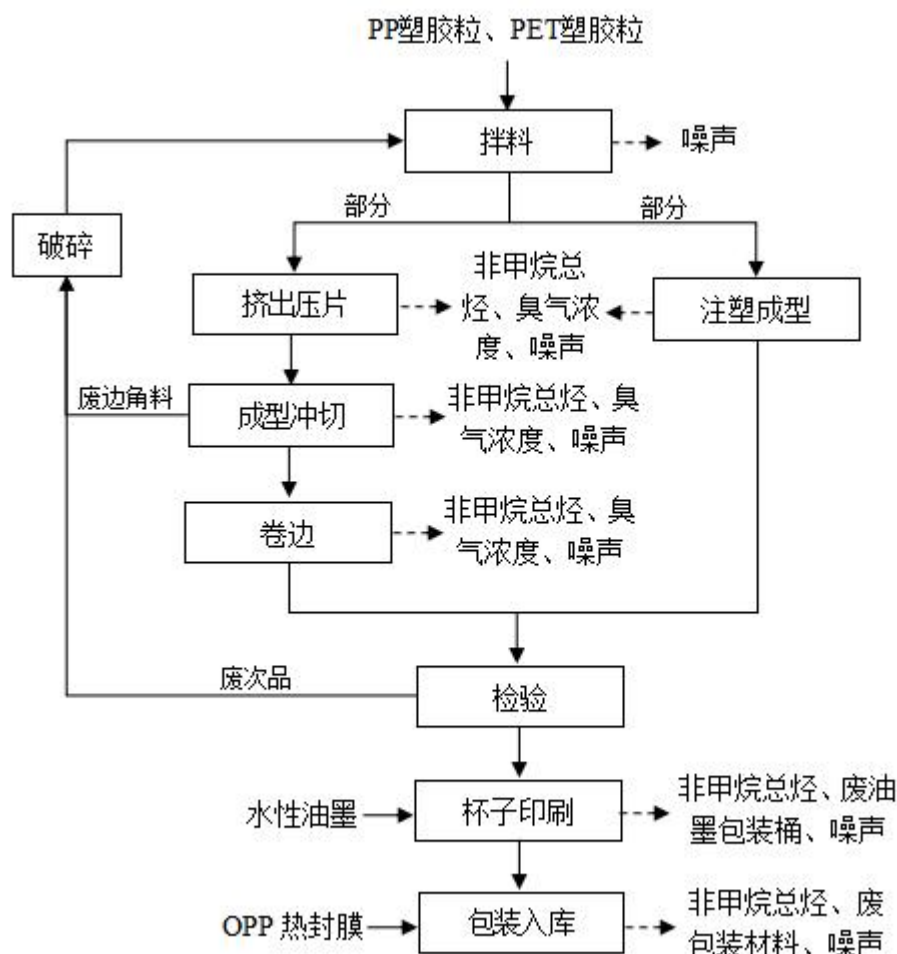
图 2-2 项目杯子生产工艺流程图
