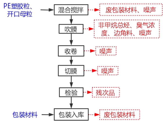
图 2-4 葫芦膜工艺流程图
