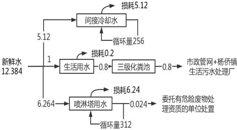
图 2-1 项目水平衡图 (t/d)
