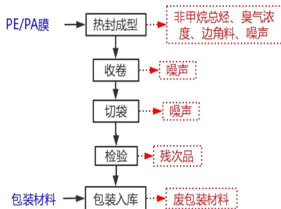
图 2-5 气柱袋工艺流程图
