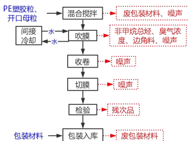
图 2-3 拉伸膜工艺流程图
