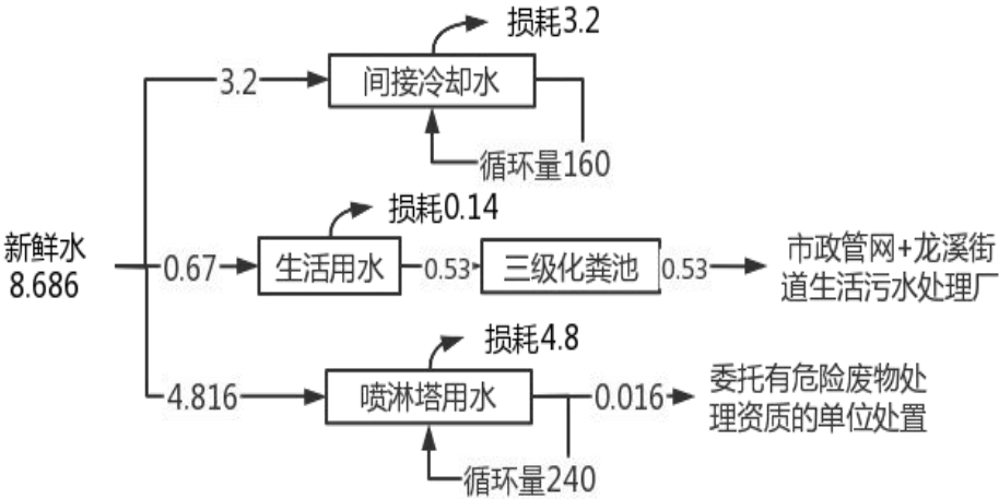
图 2-2 项目水平衡图 (t/d)
