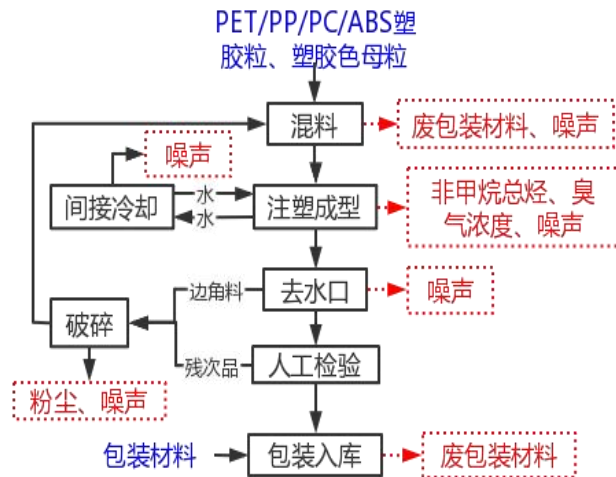
图 2-3 项目塑料零件生产工艺流程图
