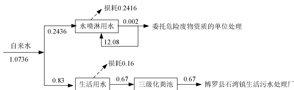
图 1 项目水量平衡图（单位：t/d）
