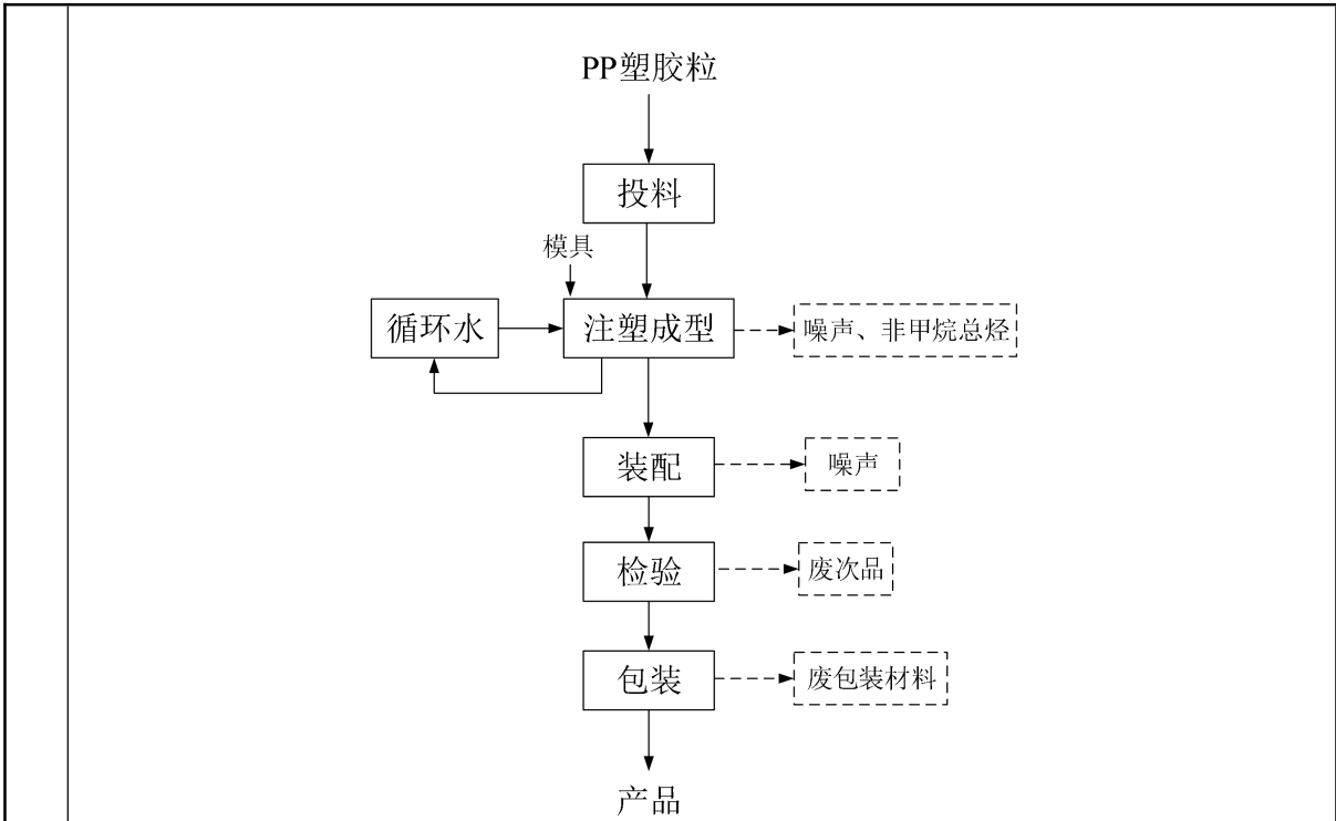
图 3 塑料配件生产工艺流程图及产污环节
