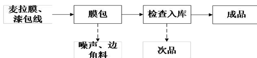
图 2-2 项目麦拉线生产工艺流程及产污环节图
