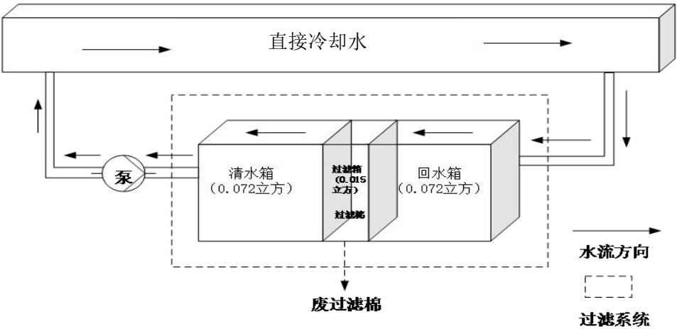
图 4-1 直接冷却水废水过滤处理系统示意图
