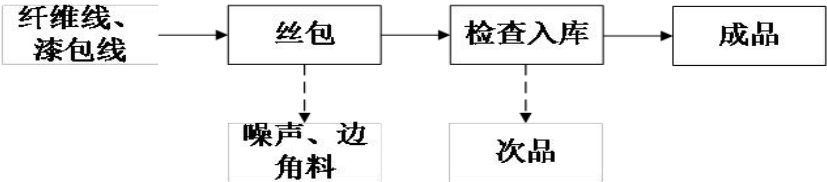
图 2-4 项目丝包线生产工艺流程及产污环节图
