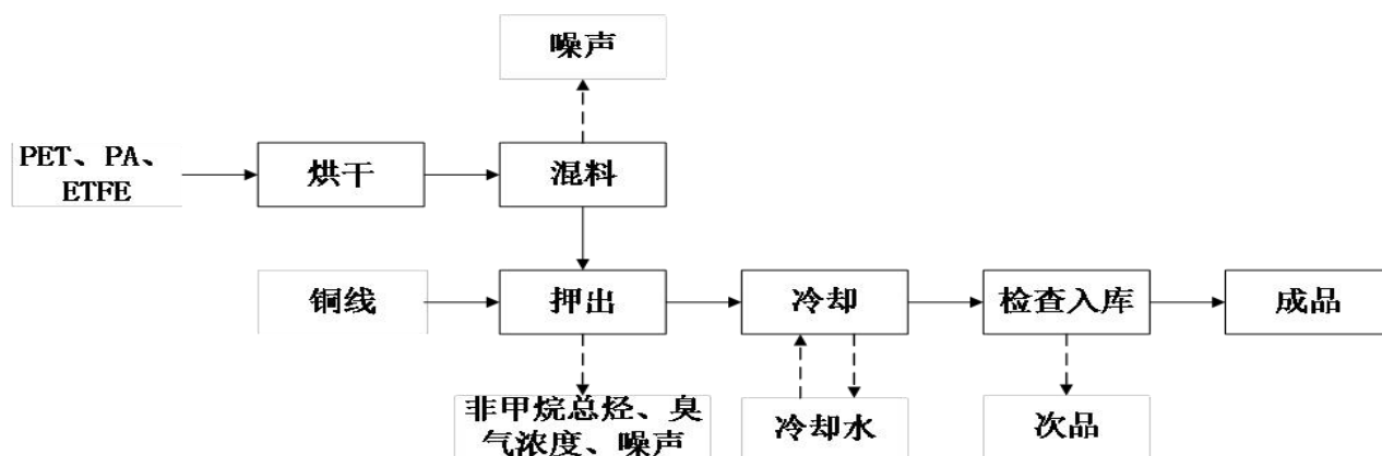
图 2-2 项目绝缘线生产工艺流程及产污环节图
