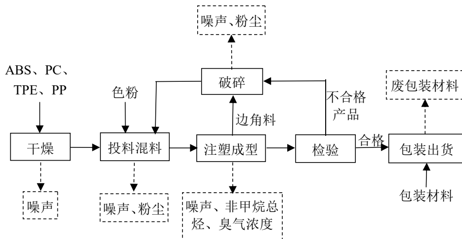
图 2-2 产品生产工艺流程图
