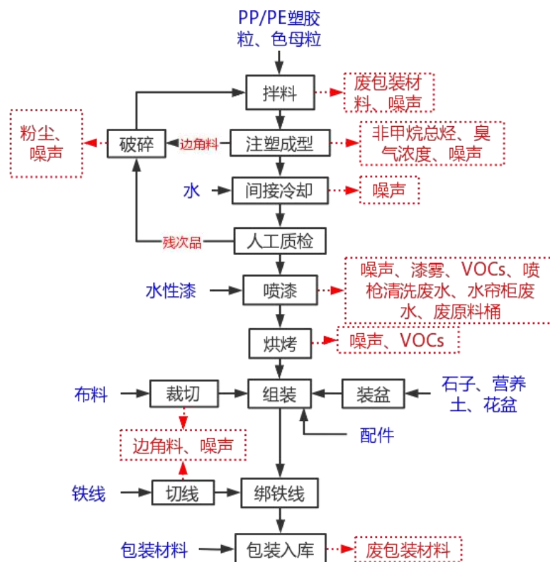
图 2-2 需喷漆仿真植物工艺流程及产污环节图
