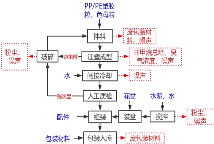
图 2-3 不需要喷漆仿真植物工艺流程及产污环节图
