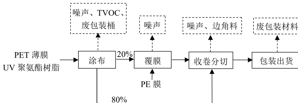
图 2-1 产品生产工艺流程图
