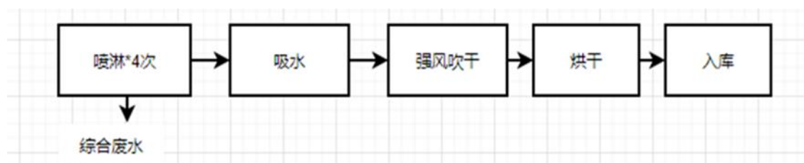
图 2-13 改扩建新增清洗线 1（用于柔性印刷单层线路板）工艺流程图
