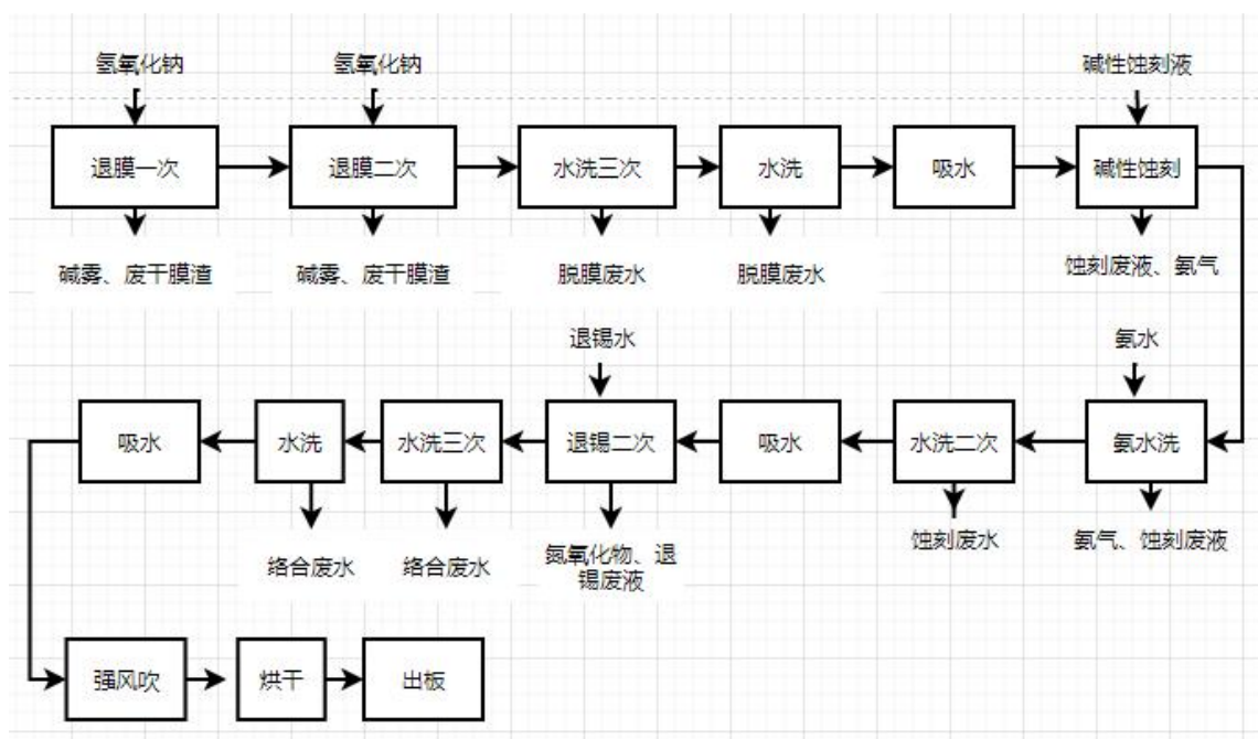
图 2-25 碱性蚀刻线工艺流程图
