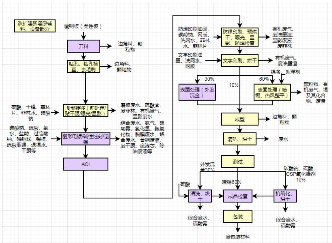
图 2-9 改扩建后项目柔性印刷单层线路板工艺流程图
