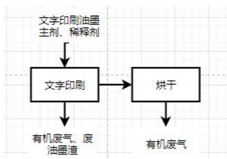
图 2-27 文字印刷工艺流程图
