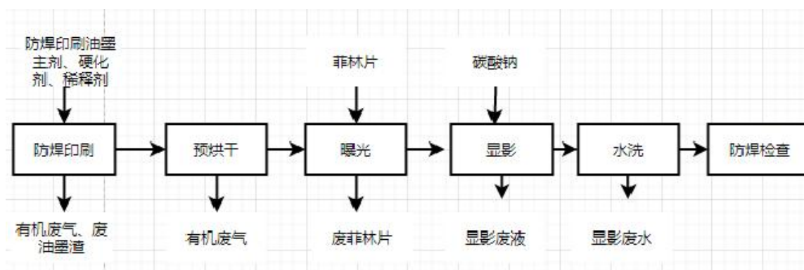
图 2-26 防焊印刷、预烘干、曝光、显影、水洗、防焊检查工艺流程图
