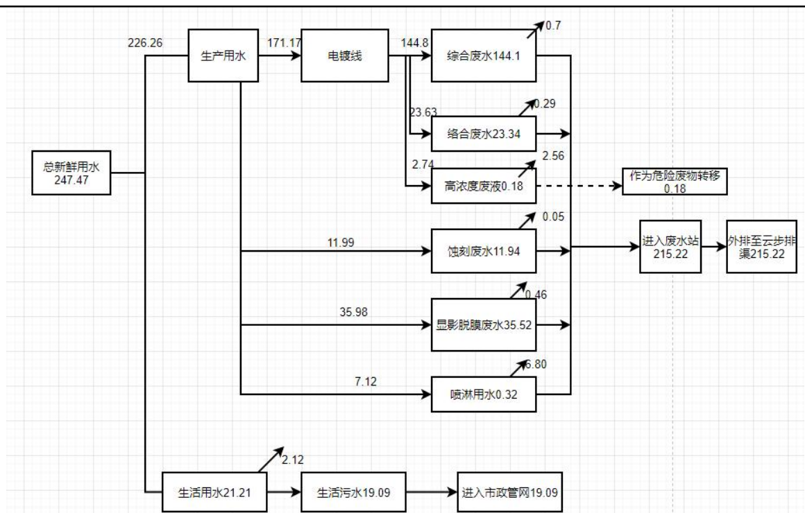
图 2-1 现有项目水平衡图 (m³/d)
