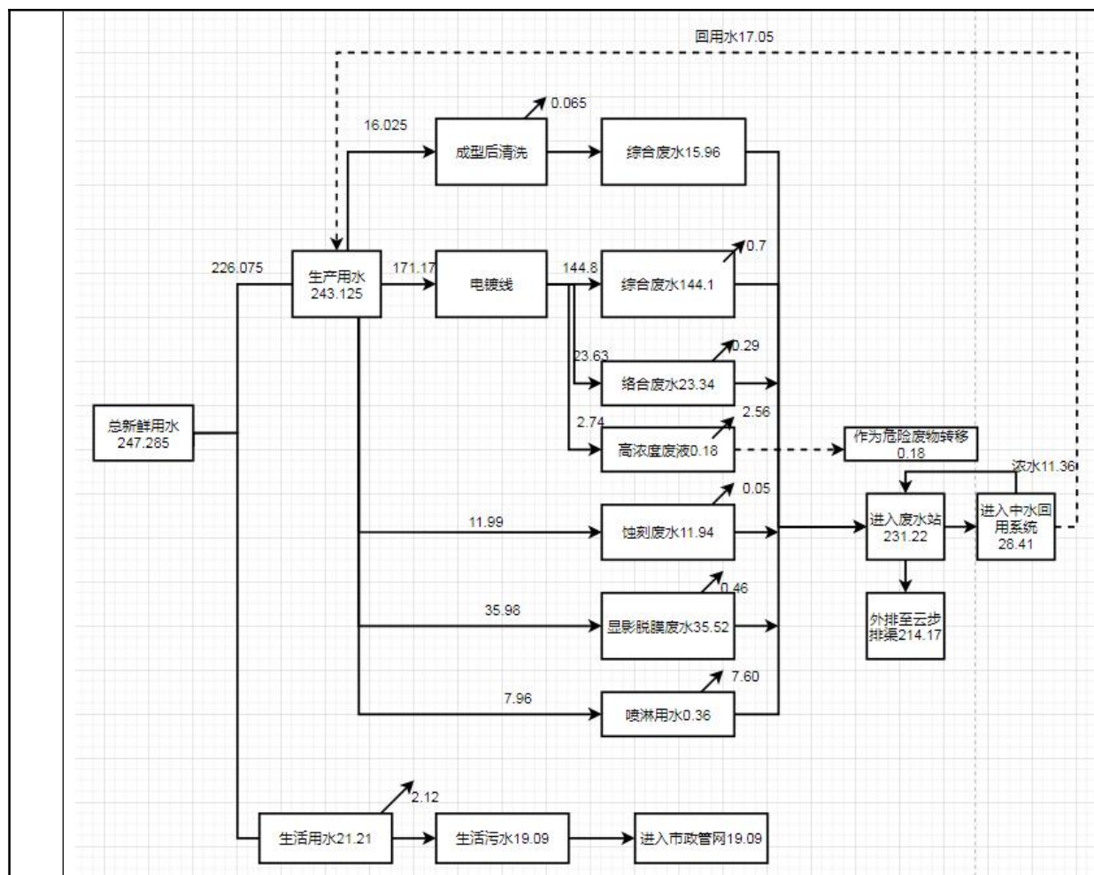
图 2-3 改扩建后项目水平衡图
