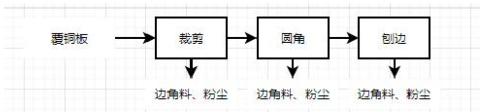
图 2-21 开料工序流程图
