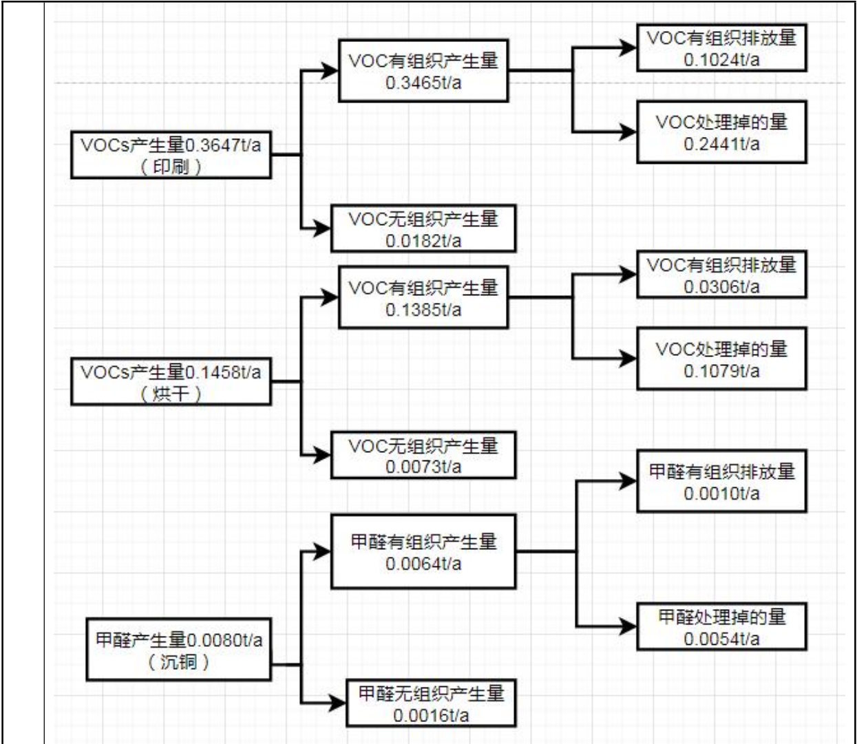
图 2-4 现有项目 VOCs 平衡图
