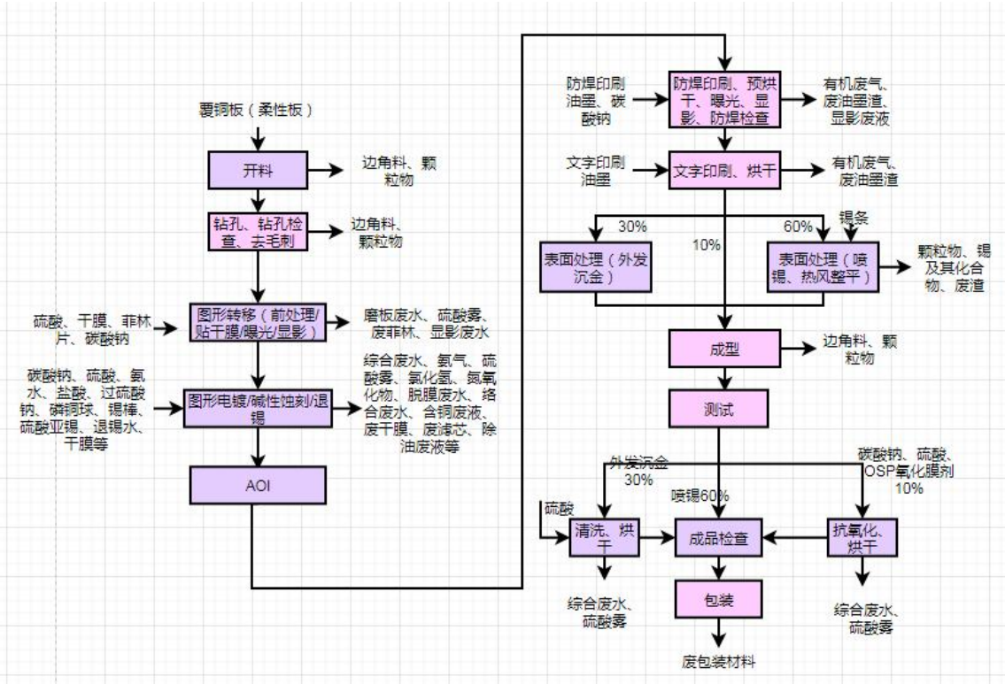
图 2-19 现有项目柔性印刷单层线路板
