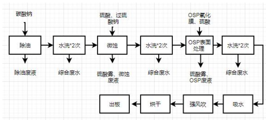
图 2-28 OSP 表面处理线工艺流程图
