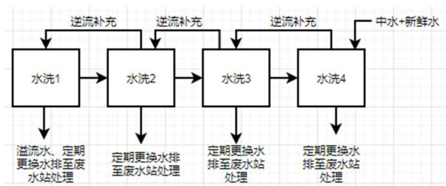
图 2-14 清洗线 1 的水洗流程图
