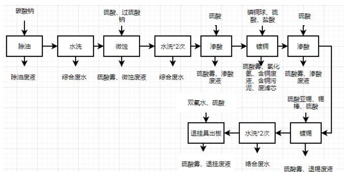
图 2-24 图形电镀线工艺流程图
