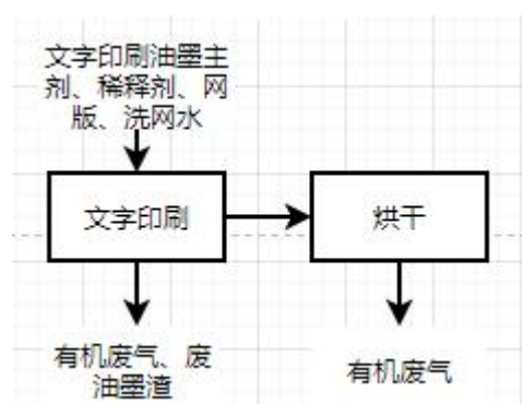
图 2-15 文字印刷、烘干工艺流程图
