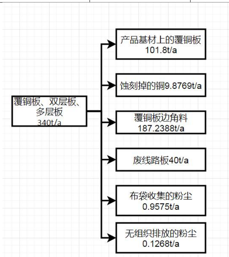
图 2-7 现有项目覆铜板物料平衡图
