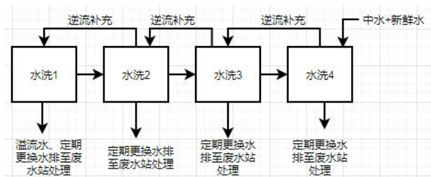
图 2-17 清洗线 1 的水洗流程图
