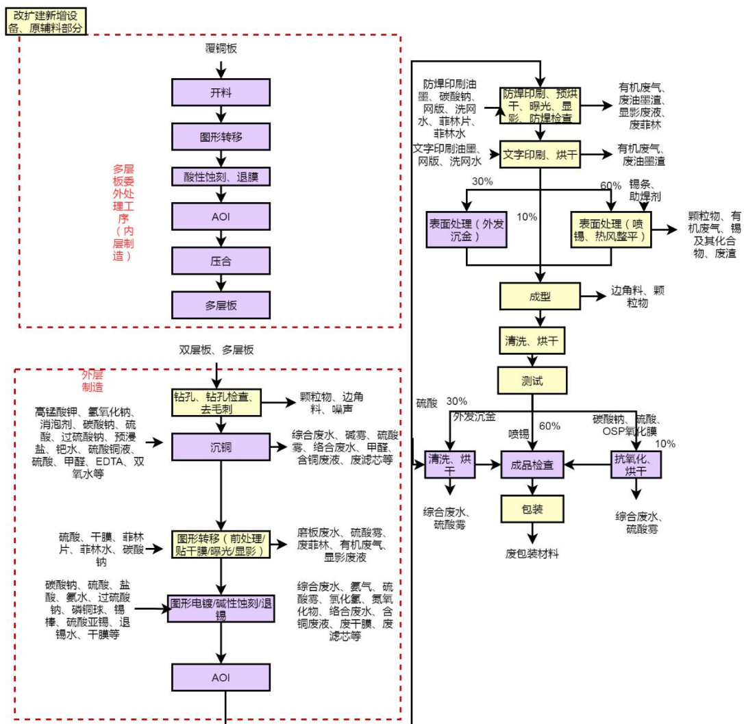
图 2-10 改扩建后项目双面板、多层板主要生产工艺流程图
