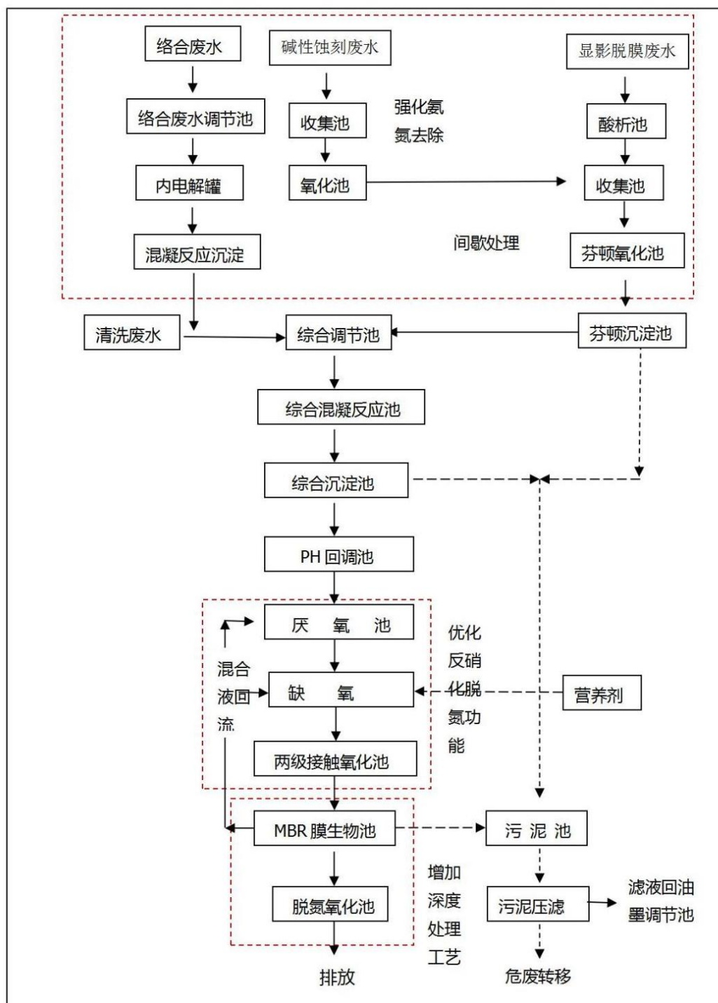
图 2-31 现有项目的废水处理工艺流程图
