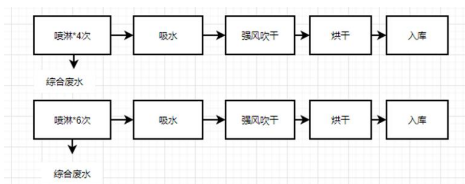
图 2-16 改扩建新增清洗线工艺流程图
