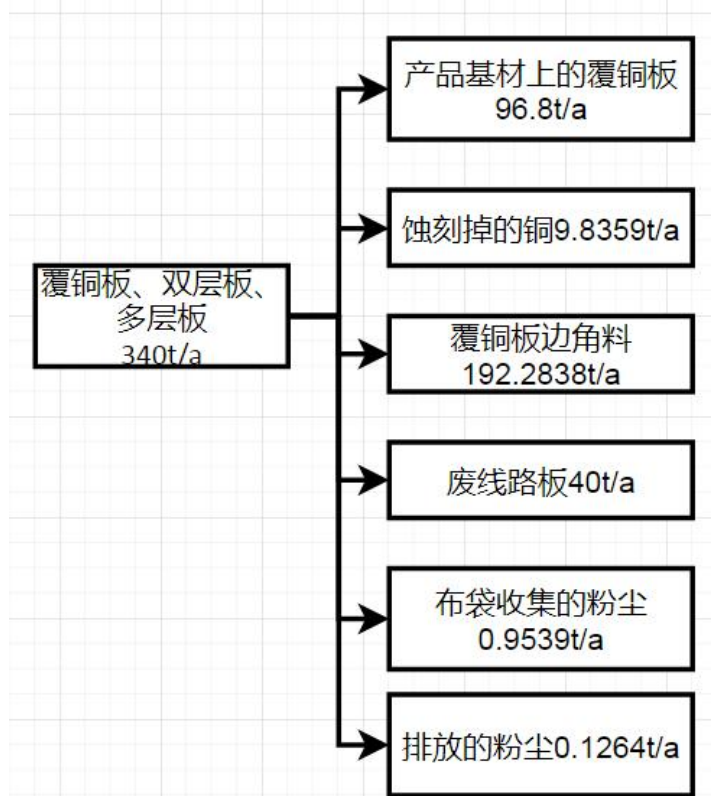
图 2-8 改扩建后项目覆铜板物料平衡图
