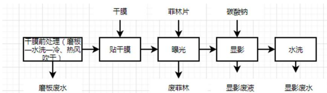
图 2-23 图形转移工艺流程图
