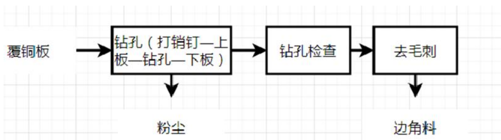
图 2-22 钻孔、钻孔检查、去毛刺流程图
