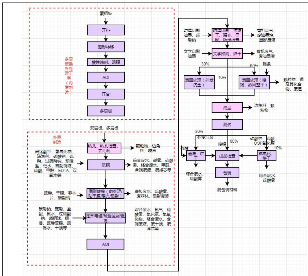
图 2-20 现有项目双面板、多层板主要生产工艺流程图
