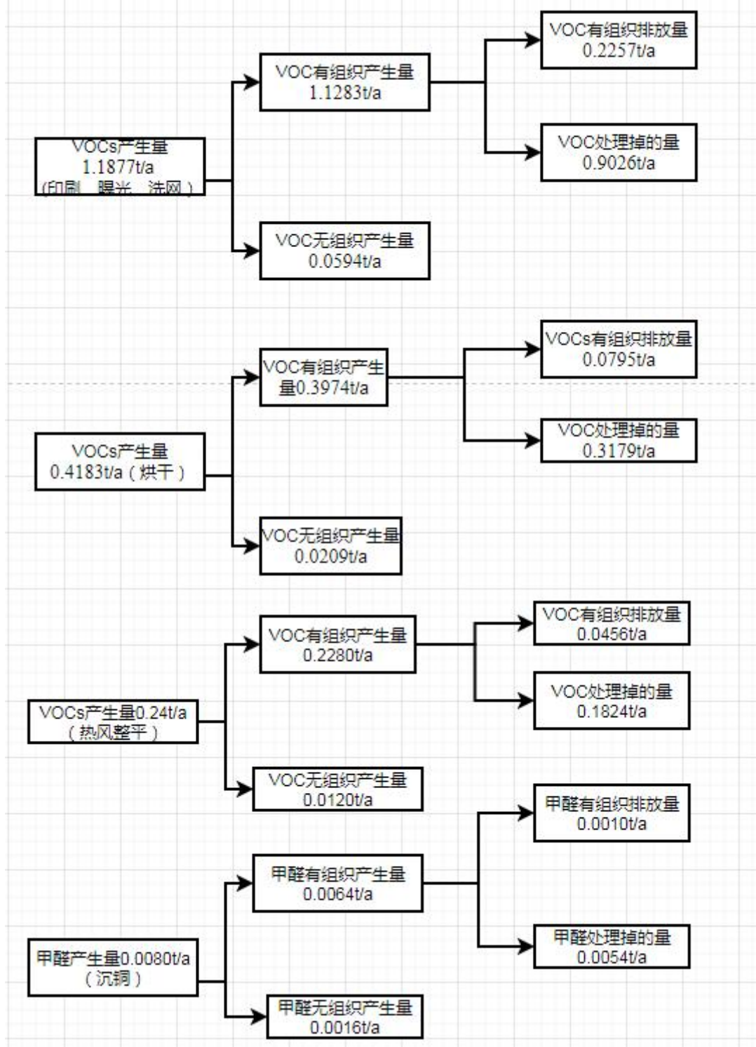
图 2-6 改扩建后全厂 VOCs 平衡图
