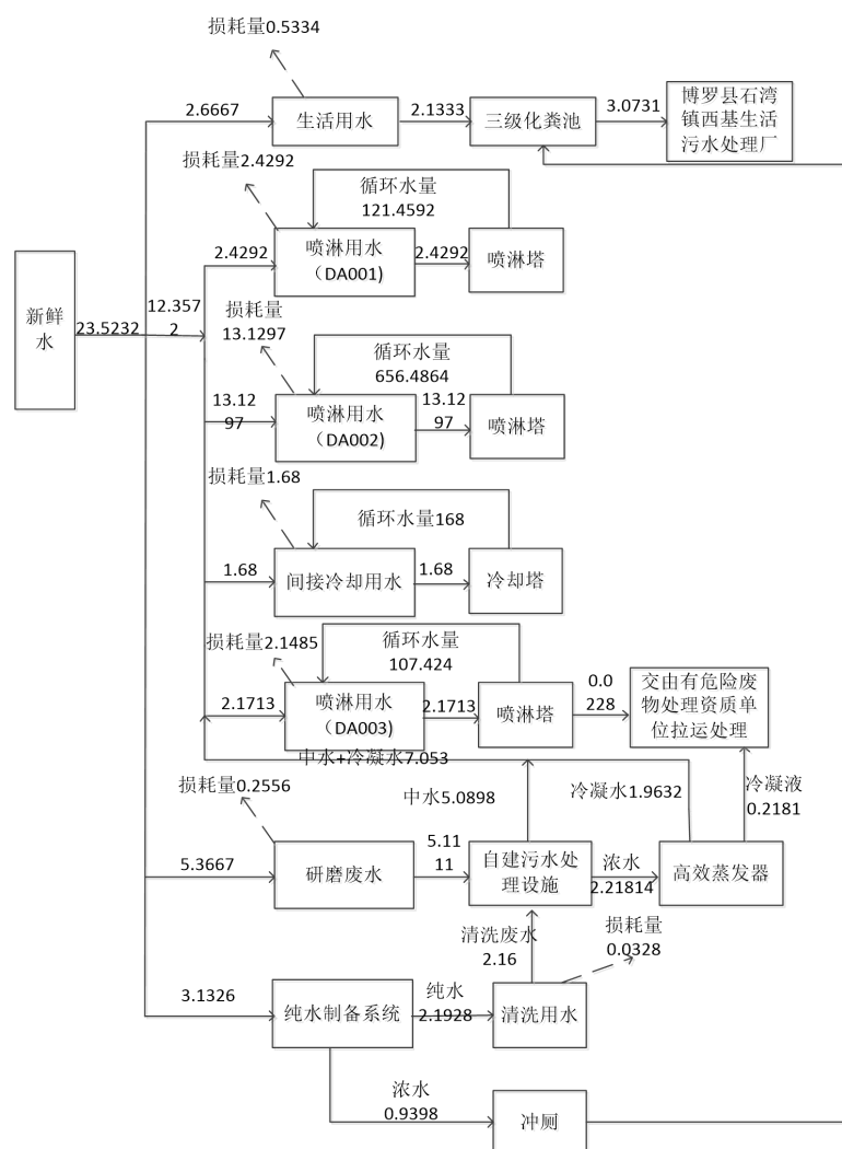
图1 改扩建后全厂项目水平衡图 (t/d)
