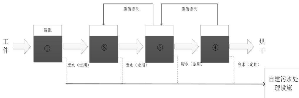
图 3 清洗工艺流程及产污节点图
