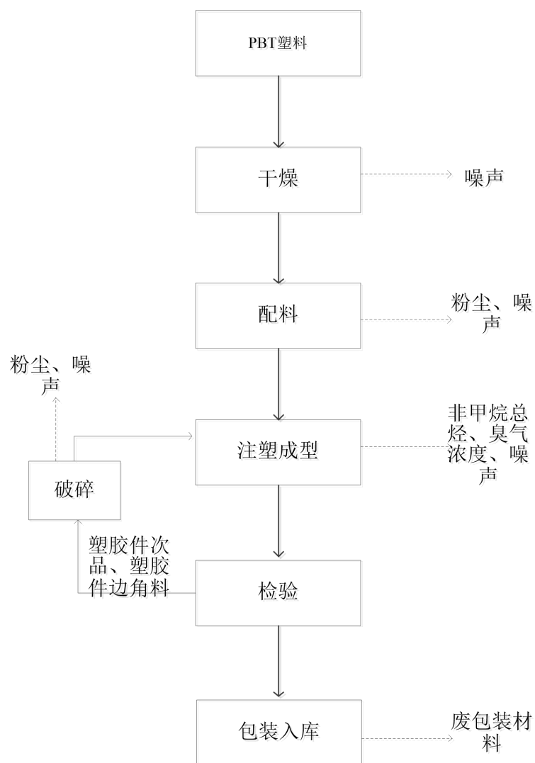
图 4 PBT 塑胶配件生产工艺流程及产污图
