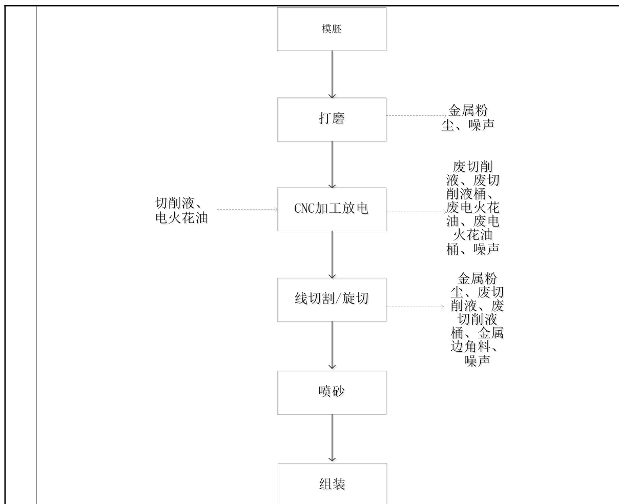
图 5 模具生产工艺流程及产污图
