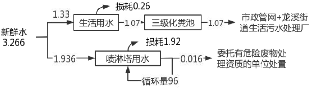
图 2-2 项目水平衡图 (t/d)
