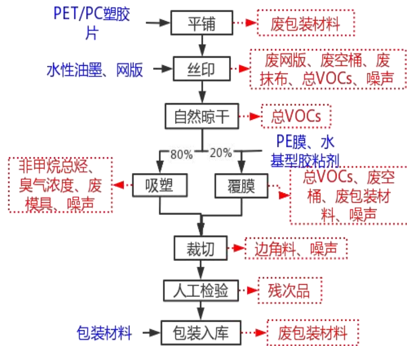
图 2-3 项目丝印胶片生产工艺流程图
