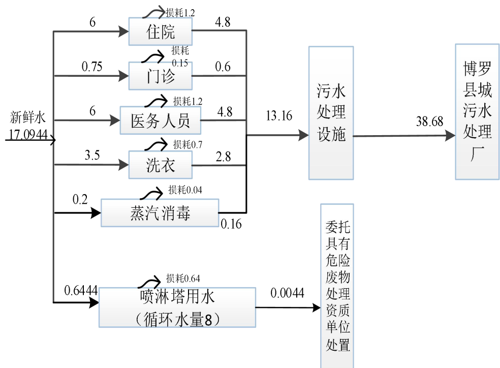
图 1 项目水平衡图（单位：t/d）
