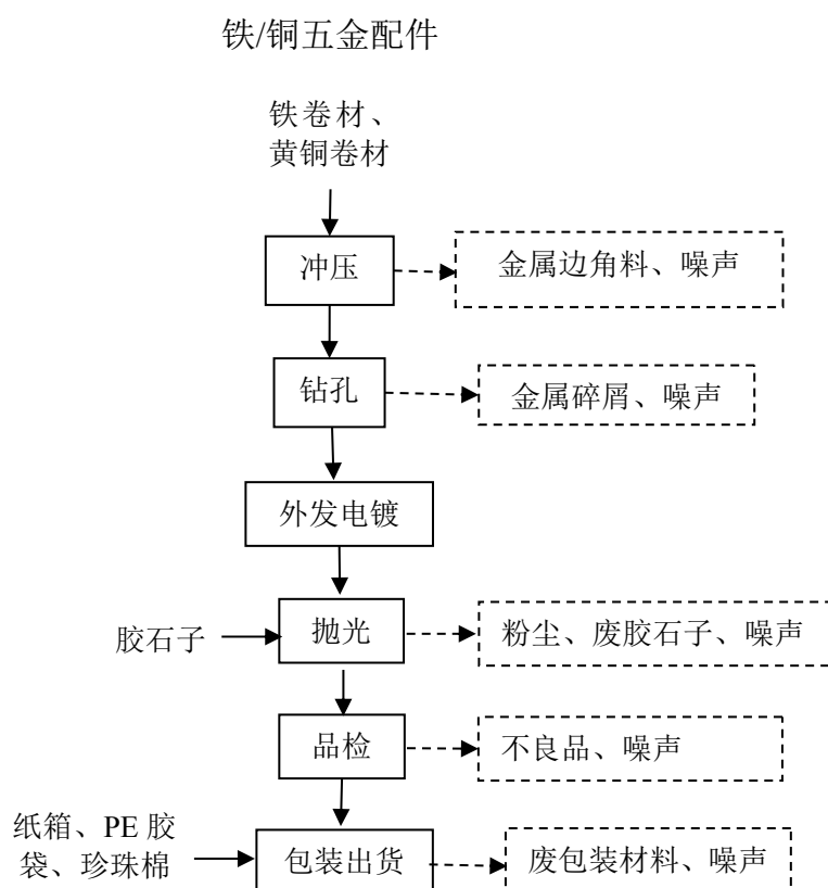
图 2-3 项目生产工艺流程图
