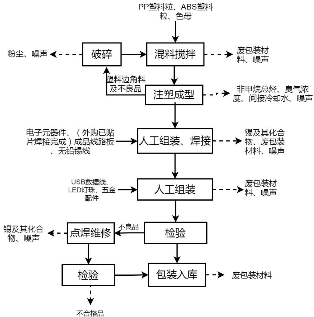
图2-2 项目的生产工艺流程图
