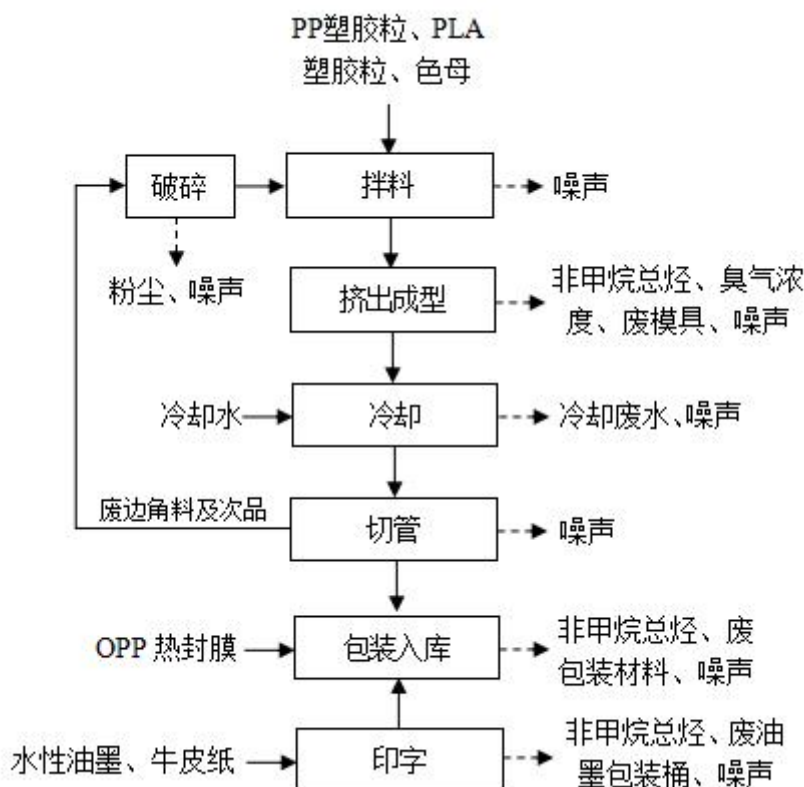
图 2-4 项目吸管生产工艺流程图
