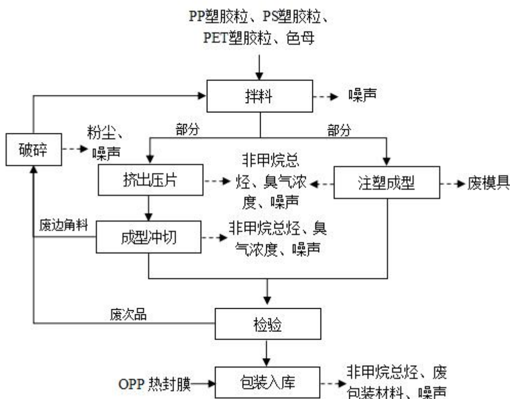
图 2-3 项目盖子生产工艺流程图
