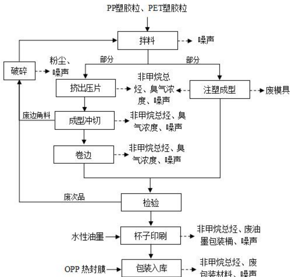
图 2-2 项目杯子生产工艺流程图
