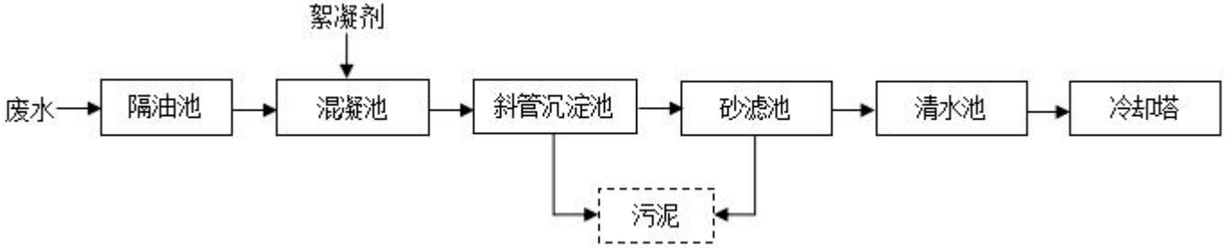
图 4-1 废水处理设施工艺流程图
