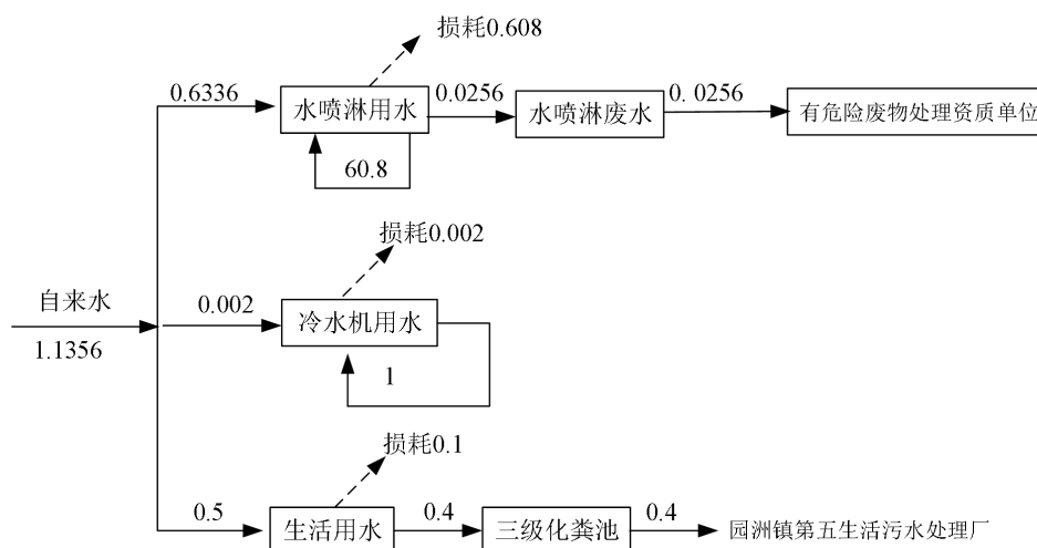
图 1 项目水平衡图 单位: \text{m}^3/\text{d}
