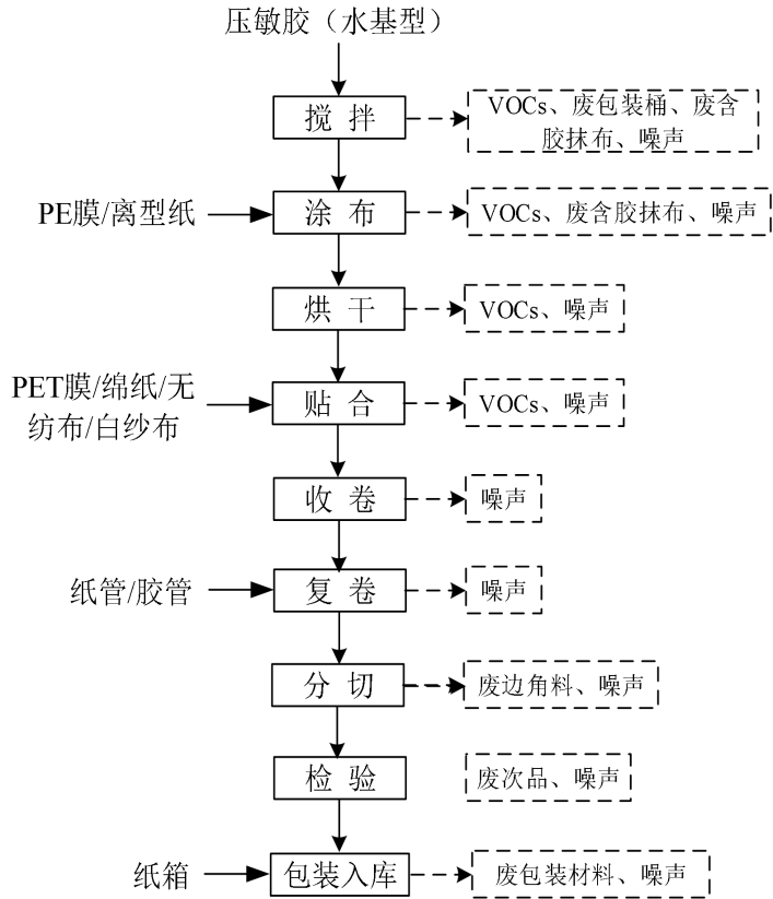
图 2 胶粘带制品生产工艺流程图 1 及产污环节
