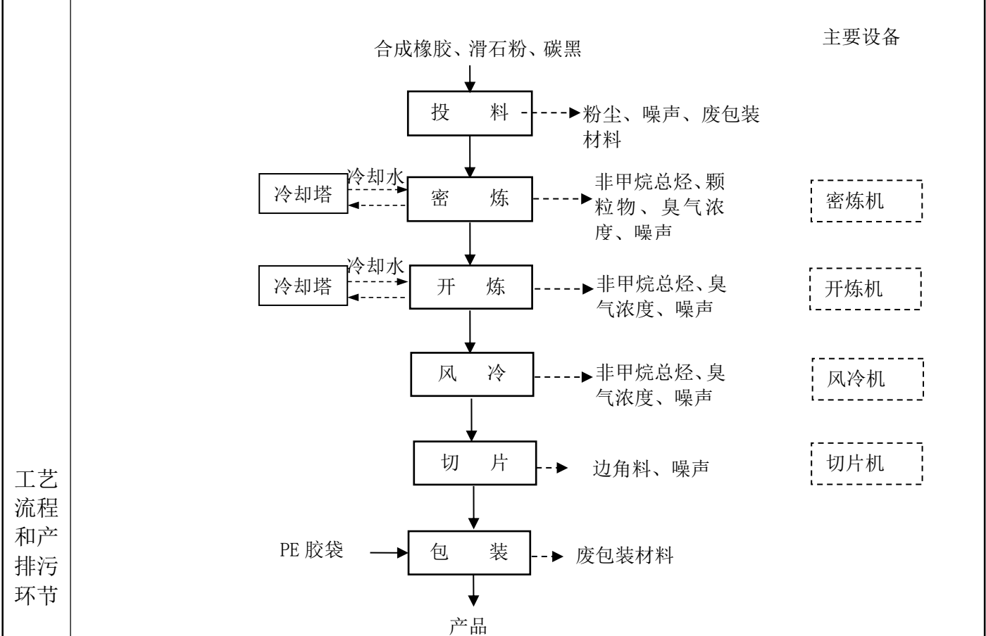
图 2-2 项目橡胶胶片生产工艺流程图
