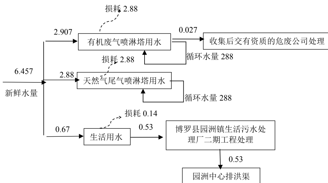
图 2-2 项目水平衡图 (m³/d)
