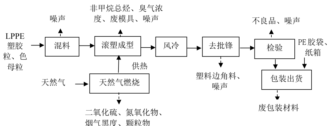
2-3 项目游戏机机壳生产工艺流程图
