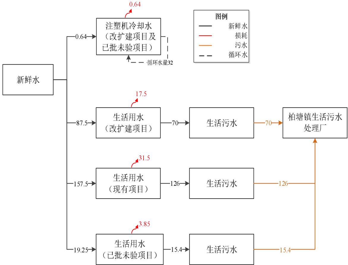
图 2.8-1 改扩建后项目总水平衡图（单位：t/d）
