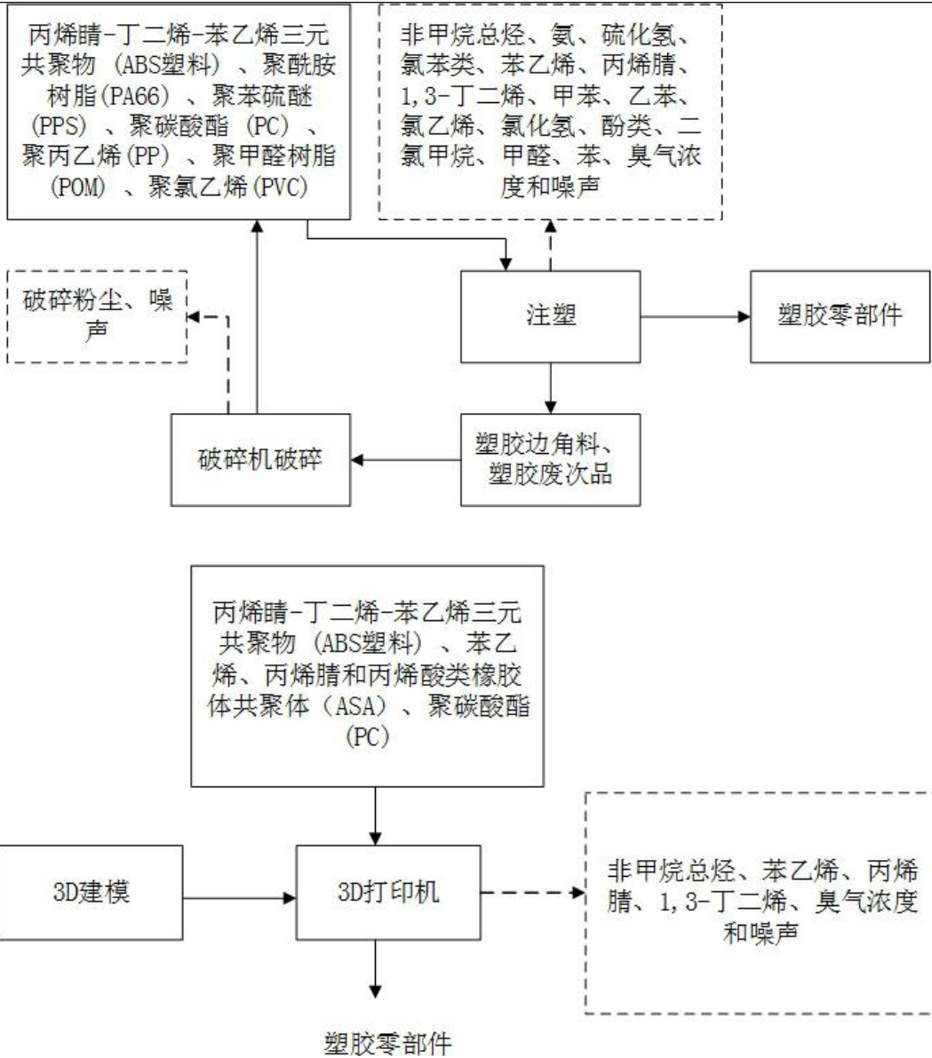
厂房一尚未建设注塑工序、3D 打印工序和破碎工序工艺流程图
