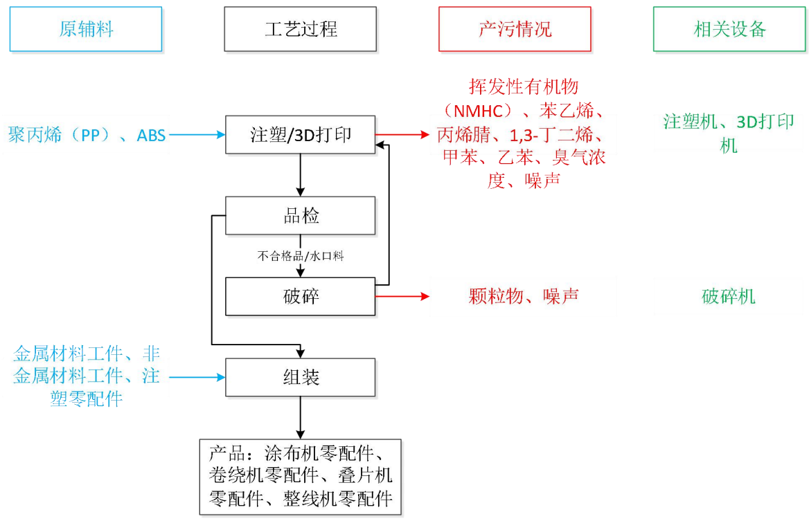
图 2.11-5 注塑加工工件生产工艺流程图
