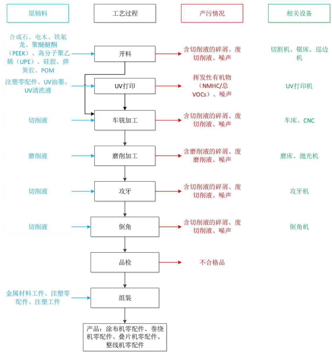
图 2.11-2 非金属材料工件生产工艺流程图
