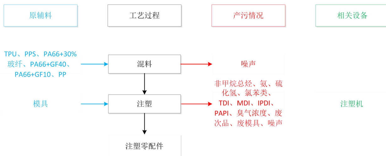
厂房二尚未建设注塑工序工艺流程图
