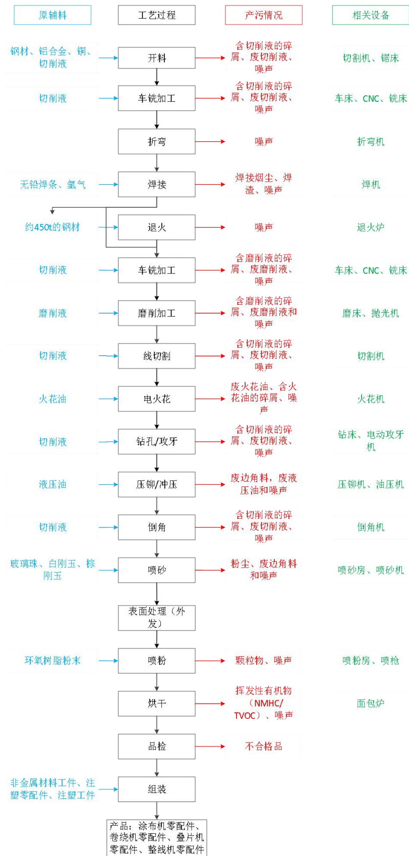
图 2.11-1 金属材料工件生产工艺流程图
