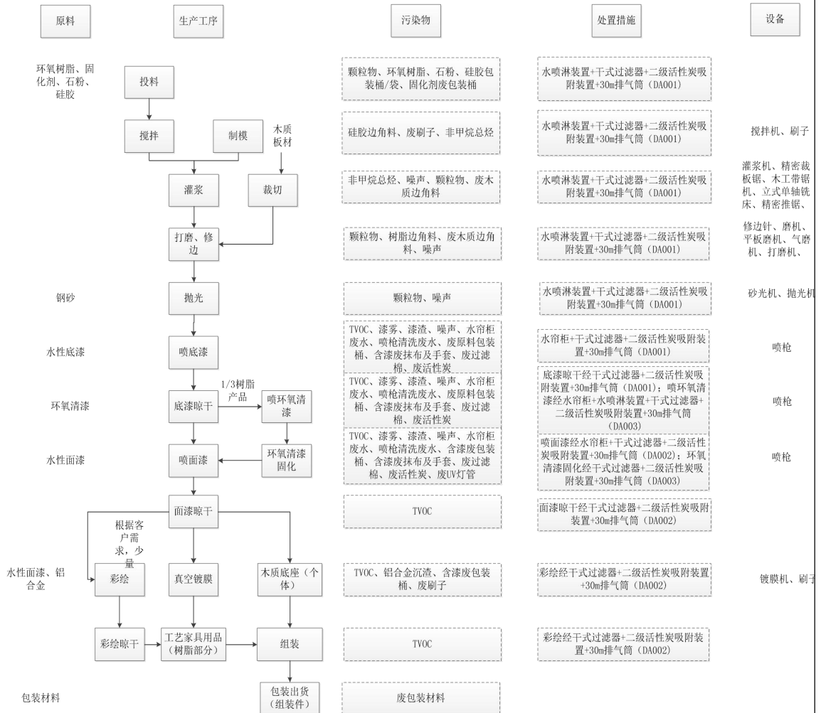
图 2-2 项目工艺家具用品工艺流程图
