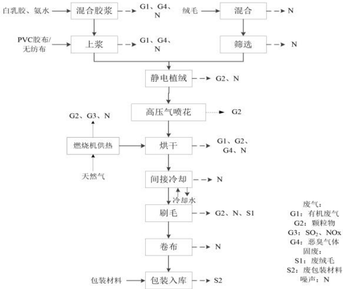
图 2-5 生产工艺流程图
