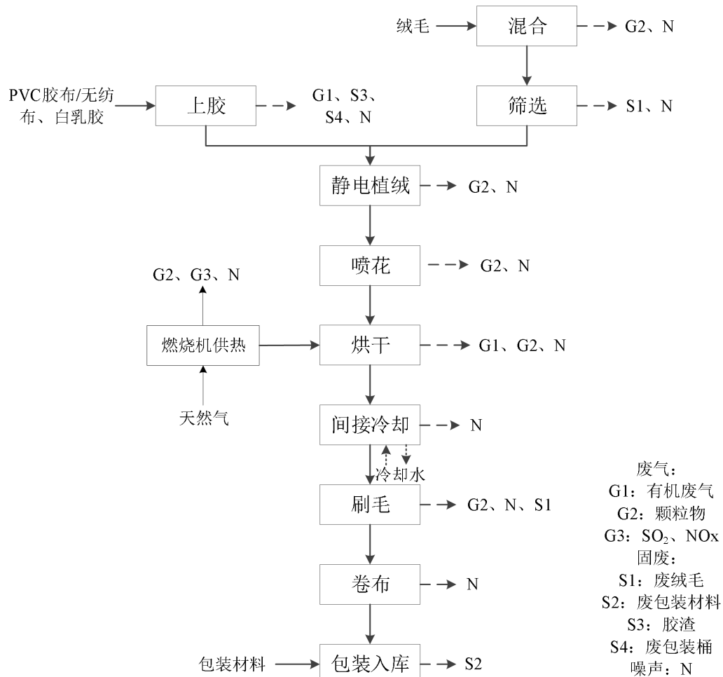
图 2-4 生产工艺流程图
