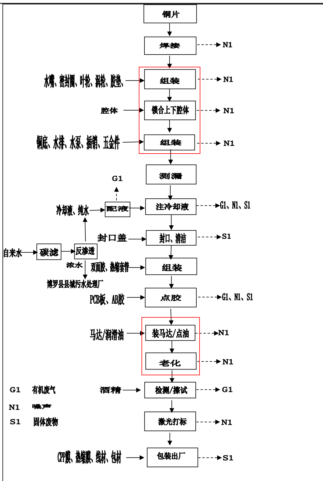
图 2-3 项目水冷散热器生产工艺流程及产污节点图
