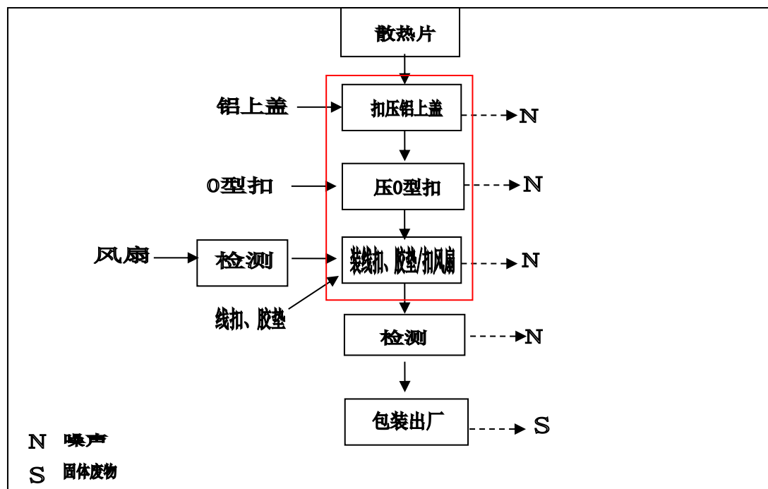
图 2-2 项目空冷散热器生产工艺流程及产污节点图
