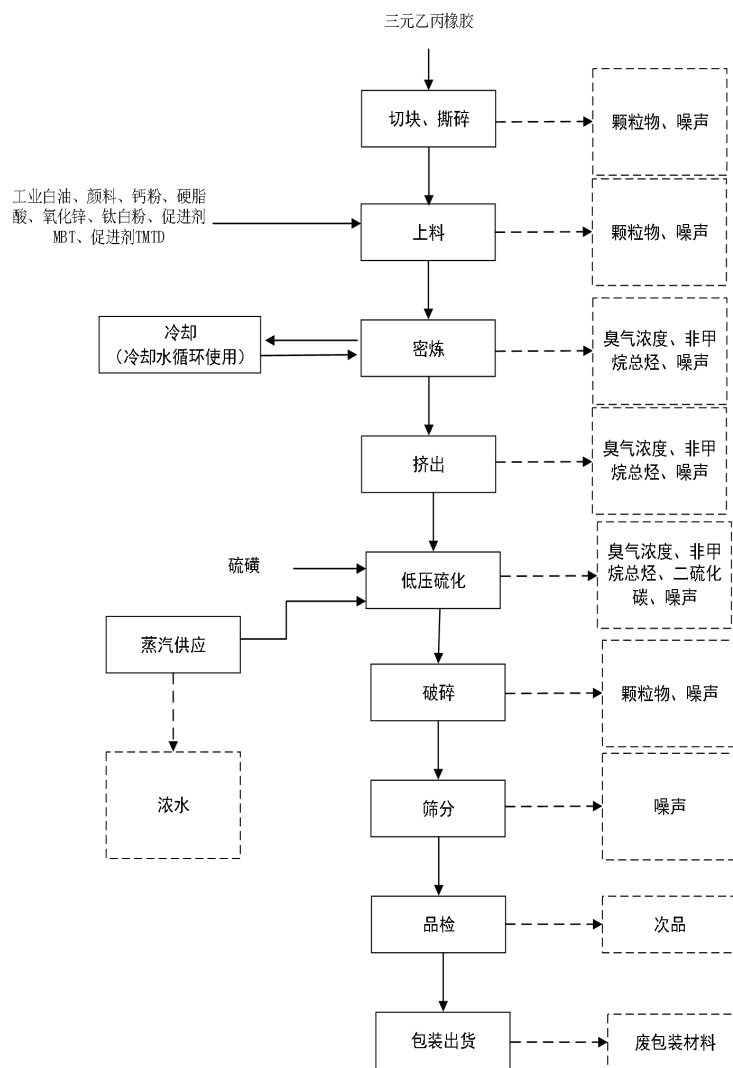
图 2-4 现有项目生产工艺流程图
