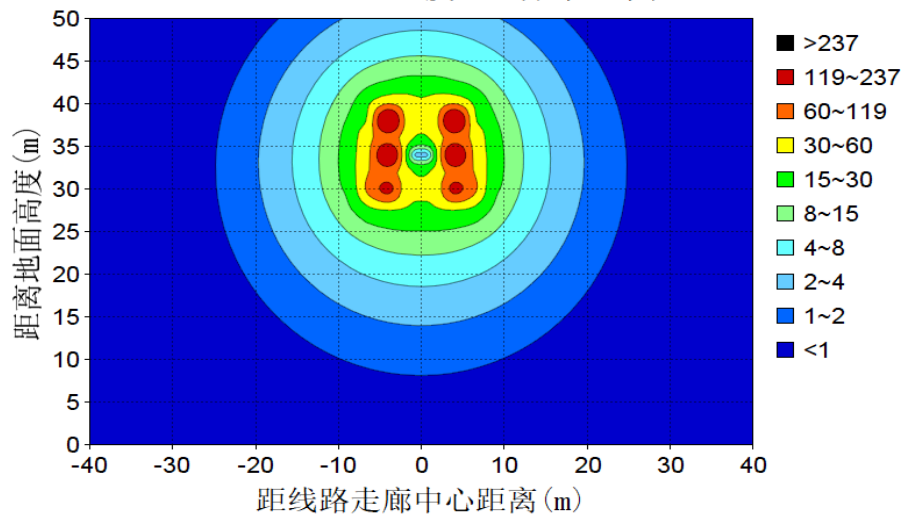
图 5-1 线路 I 四回段段拟选最不利塔型磁感应强度随距离变化图 工频磁感应强度空间分布 单位：μT
