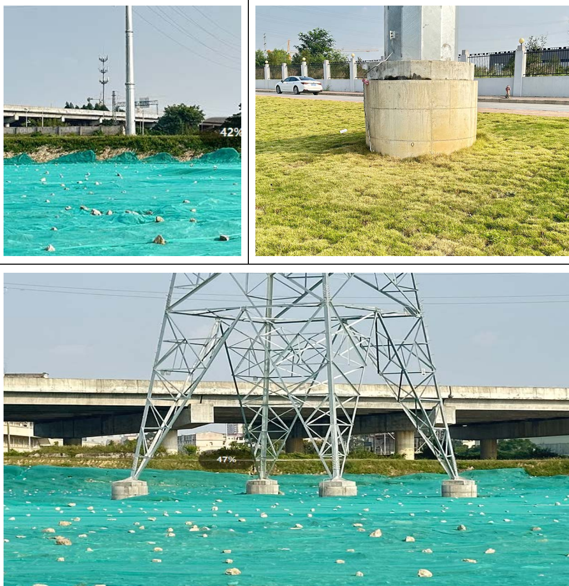
图 4-1 建设线路施工完毕后现场照片
