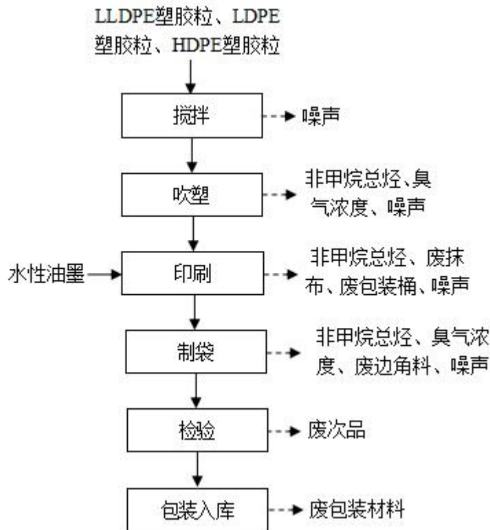
图 2-3 项目塑料袋生产工艺流程图
