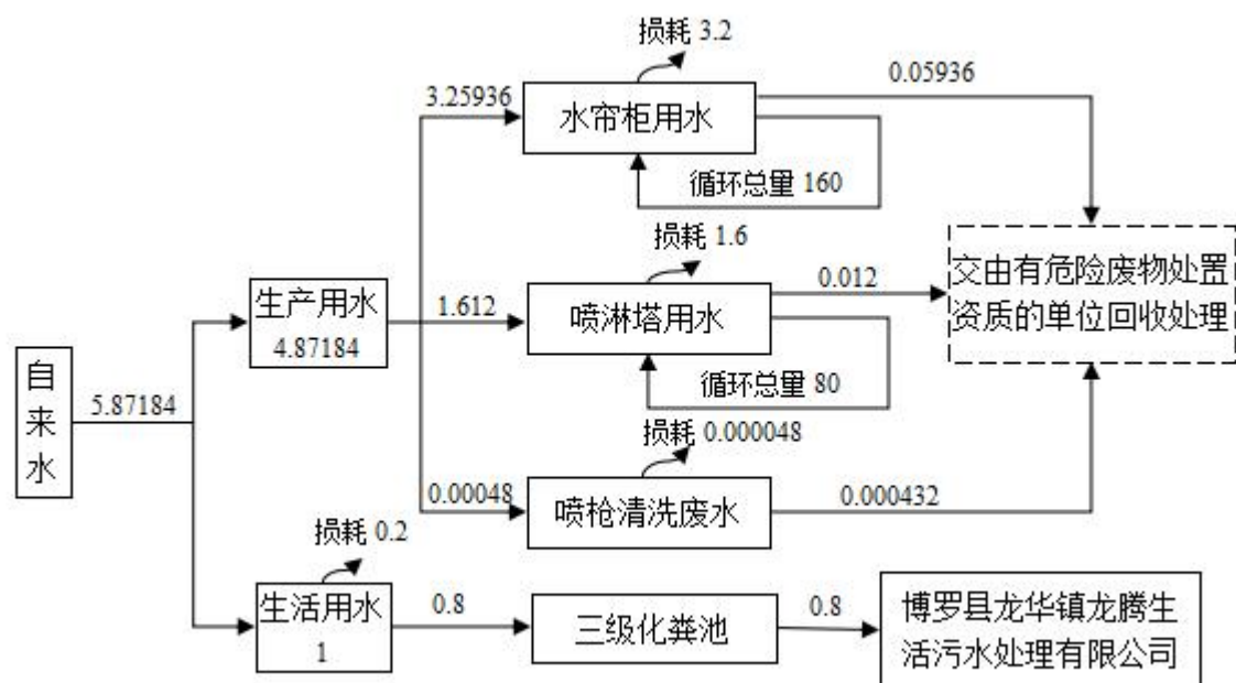
图 2-8 项目水平衡图 (t/d)
