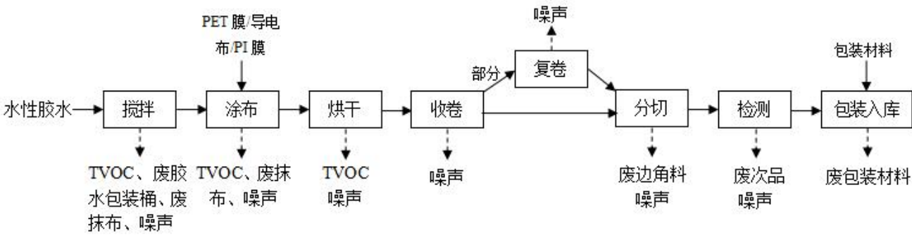
图 2-3 项目 PET 胶带、导电布胶带、PI 胶带生产工艺流程图
