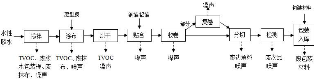
图 2-4 项目铜箔胶带、铝箔胶带生产工艺流程图
