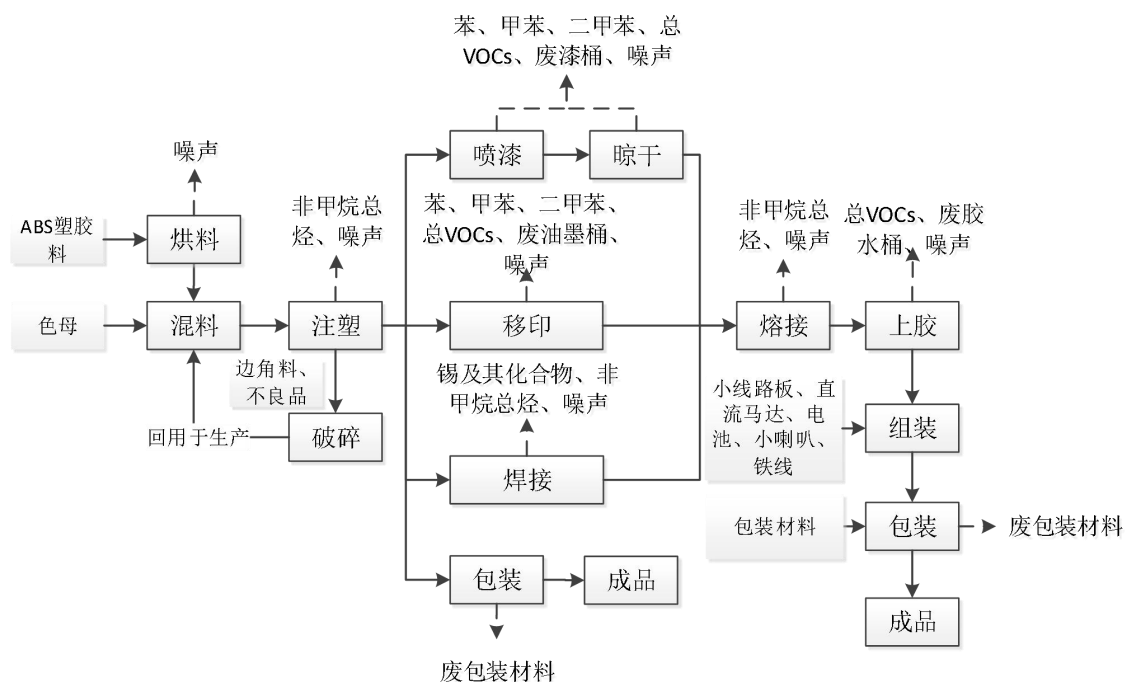
图 2-4 现有项目塑胶玩具生产工艺流程图
